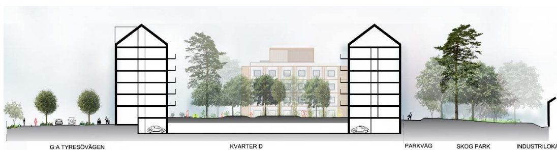
Tvärsektion genom planområdet vid kvarter D
