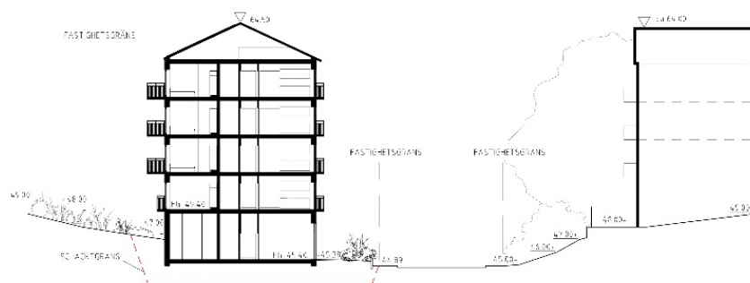
STUDENTHUSET A-A SKALA 1:200
