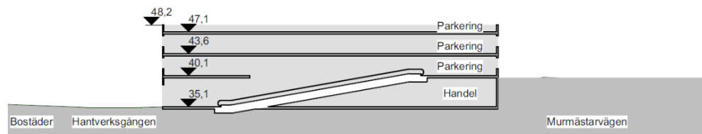
Schematiska sektioner på ny handelsbyggnad med handel i bottenplan, samt parkering och biluppställningsytor för närliggande bilhandel i flera plan. Illustration Ettelva Arkitekter
