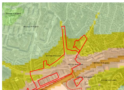
NO 2 /dygn. Orange färg redovisar ytor med halter nära gränsvärdet.
