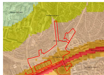
PM 10 /dygn, Röd färg markerar ytor där gränsvärdet överskrids.
