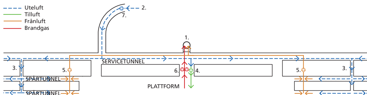
Figur 50. Principflödesschema Ventilation. Förklaringar: 1. Schakt för brandgas och frånluft, 2. Uteluftsintag (galler), 3. Tvärtunnel för uteluft till spårtunnlar, 4. Tilluftsfläkt för plattformsrum, 5. Frånluftsfläkt för spårtunnel, 6. Brandgasfläktar för plattformsrum, 7. Fläkt för ventilation och övertrycksättning av servicetunnel.
