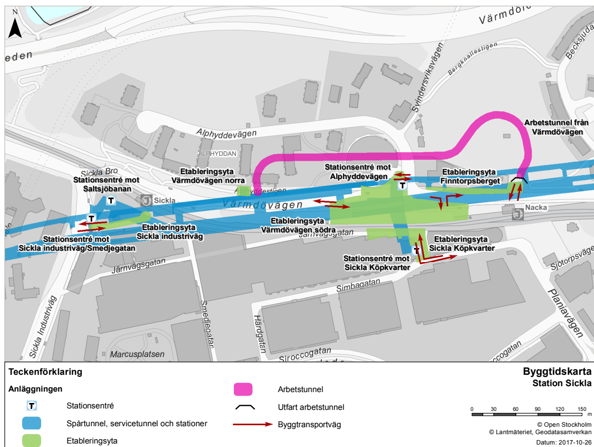
Figur 24. Etableringar för station Sickla.
