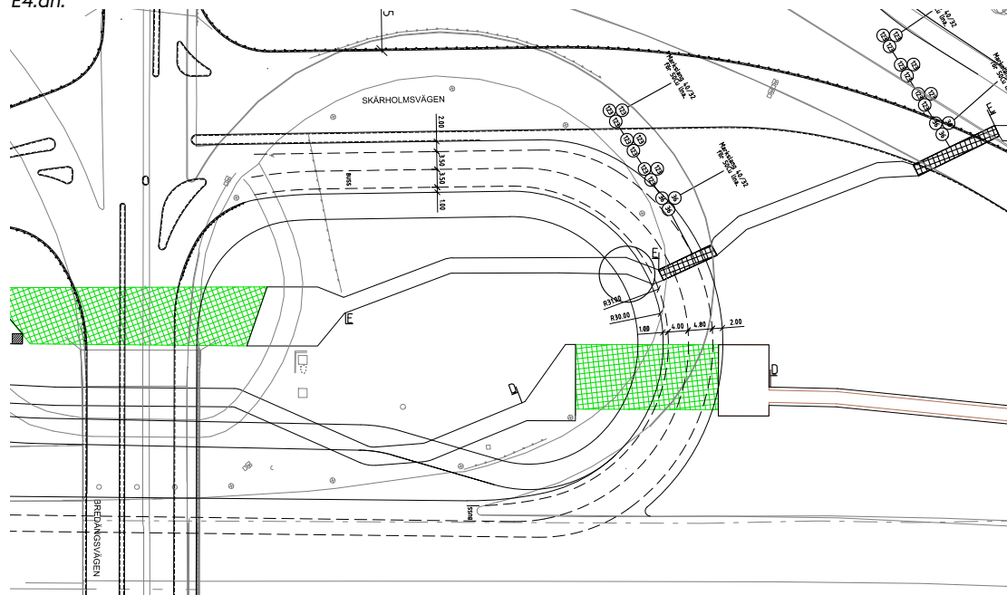
Figur 15. Busskörfält påfartsramp över högspänningsledningar som är förstärkta men med intrång på genomgående körfält på E4:an.
