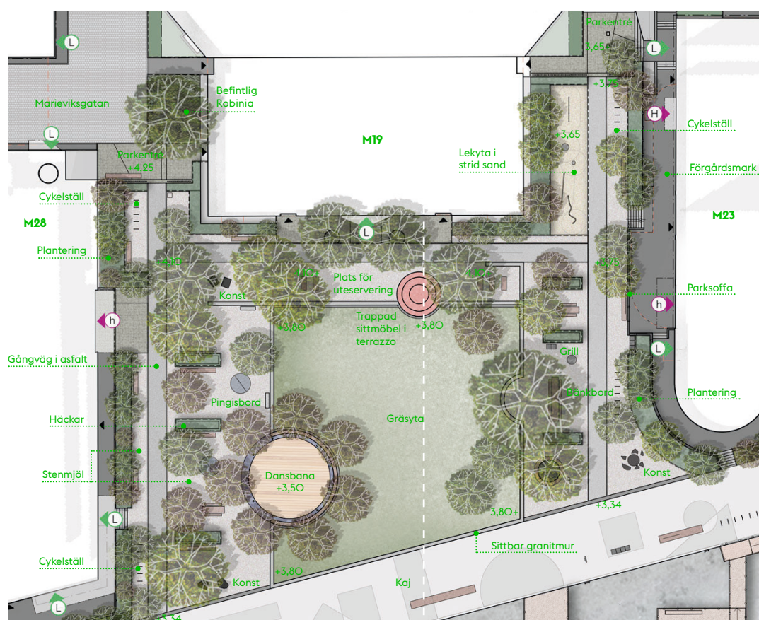
Illustrationsplan Södra parken (AJ landskap)
