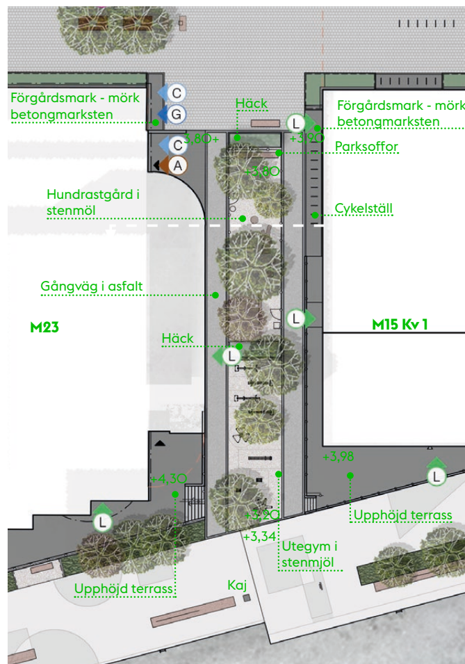
Illustrationsplan Aktivitetsparken (AJ landskap)
