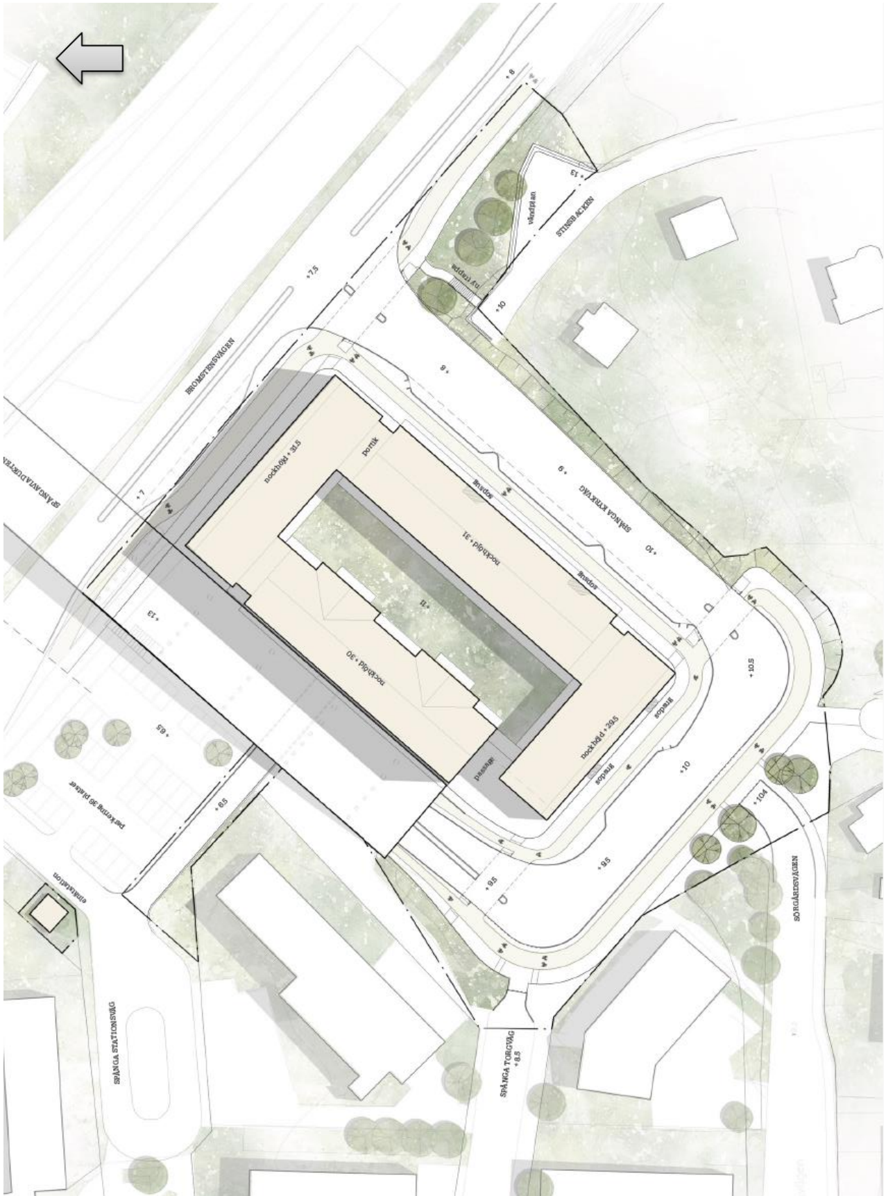
Skiss över planförslaget med Spånga Kyrkvägs nya sträckning och bebyggelseförslaget (Nivå Landskapsarkitektur).
