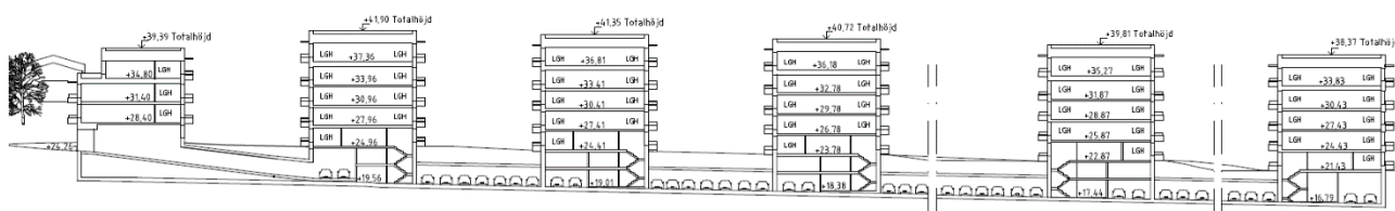
Längdsektion genom förslag på garage som försörjer området med parkeringsplatser. (Nyréns)
