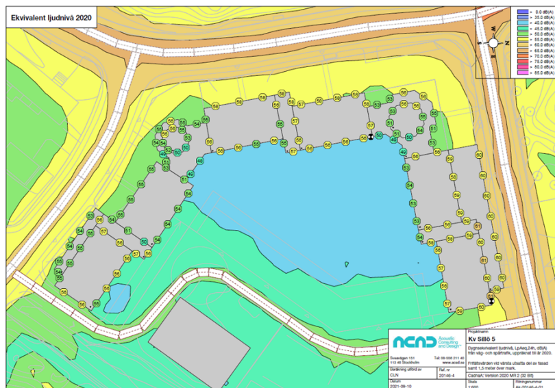
Dygnskvivalent ljudnivå från väg- och spårtrafik år 2020, befintlig bebyggelse. Ljudnivå 1,5 meter över mark (Karta: ACAD).
