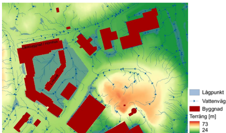
Avrinningsvägar och lågpunkter för befintliga förhållanden i övre bild och för det nya planförslaget i nedre bild. (Bild: Kragh Berglund, Structor)
