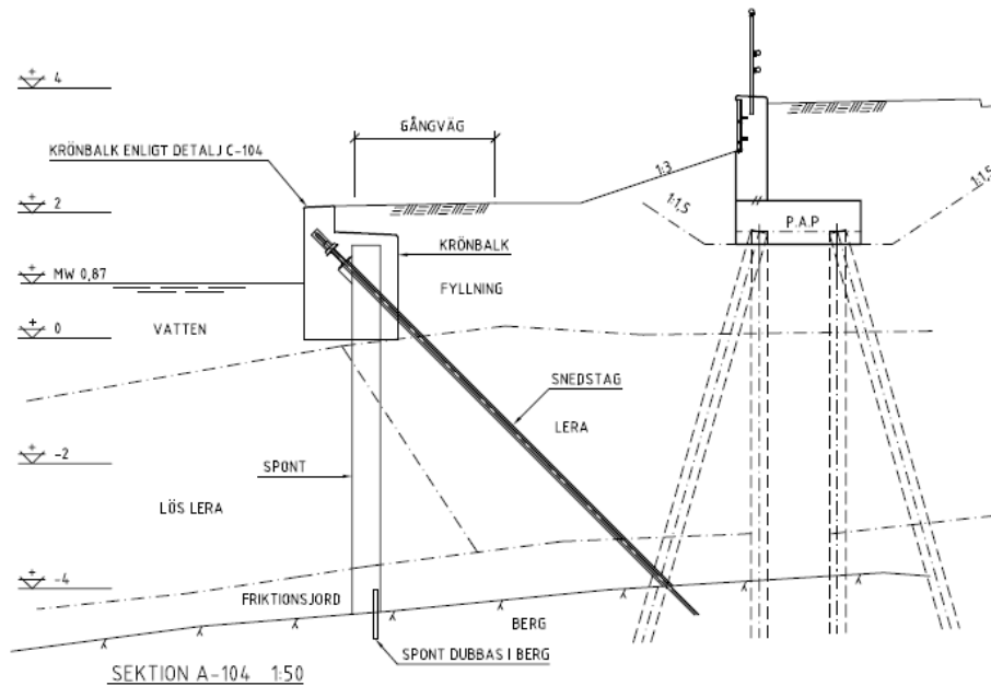
Figur 2. Arbetskiss på bakåtförankrad spont med krönbalk.
