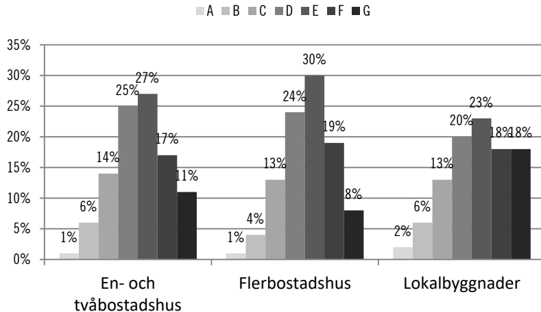
Figur 6.3 Fördelning energiklasser
