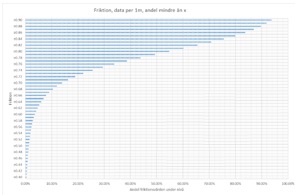
Figur 10. Andel friktionsvärden (per 1 meter) under en given friktionsnivå på vägar i bruk (Lundberg med flera, 2015).
