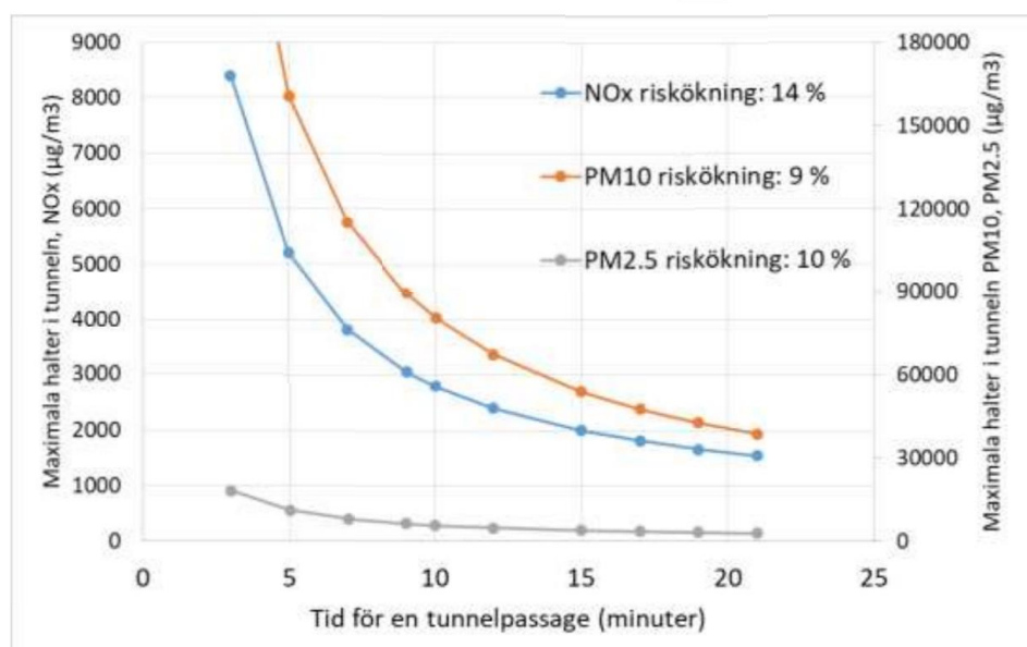
Figur 6. Maximala halter som kan accepteras någonstans i tunneln 84 med olika tider för en fordonspassage med antagande om 2 passager per dag och 220 pendlingsdagar. Baseras på att halten övrig tid är genomsnitt för gatumätningar i Stockholm år 2019 ( \text{NO}_x 12 \mu\text{g}/\text{m}^3 , \text{PM}_{10} : 23 \mu\text{g}/\text{m}^3 ; \text{PM}_{2.5} : 6 \mu\text{g}/\text{m}^3 ) och att ventilationsfiltret tar bort 95 %, 50 % och 0 % av \text{PM}_{10} , \text{PM}_{2.5} respektive \text{NO}_x . (Johansson & Forsberg, 2020)
