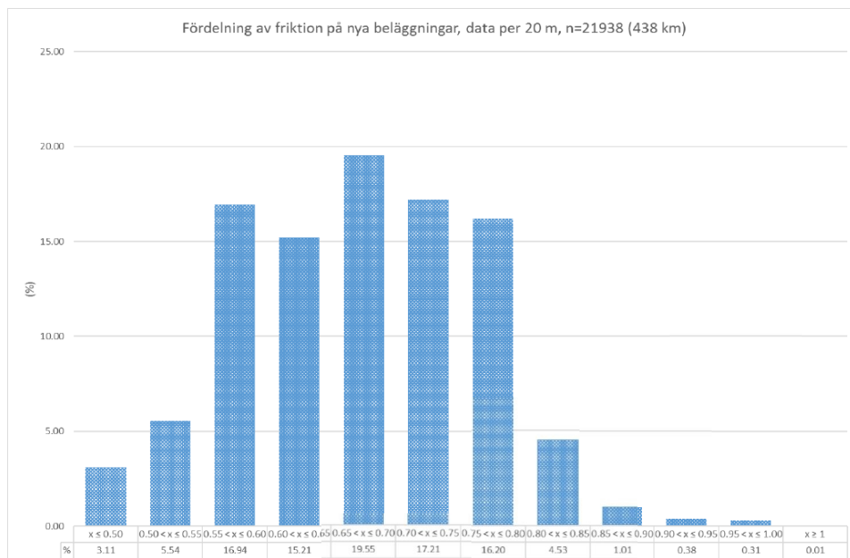
Figur 8. Normalnivåer för våtfriktion på nya beläggningar, data per 20 meter (Arvidsson, et al., 2019).
