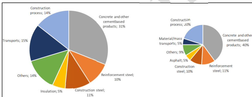
Figur 4. Emissioner av CO 2 från byggande av byggnader 7,6 miljoner ton CO 2 , respektive transportinfrastruktur 1,9 miljoner ton CO 2 (Karlsson, et al., 2020).
