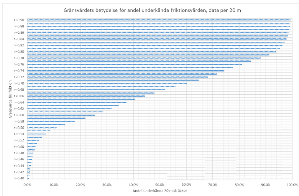
Figur 9. Andel underkända 20 metervärden vid ett förändrat gränsvärde hos nya beläggningar.
