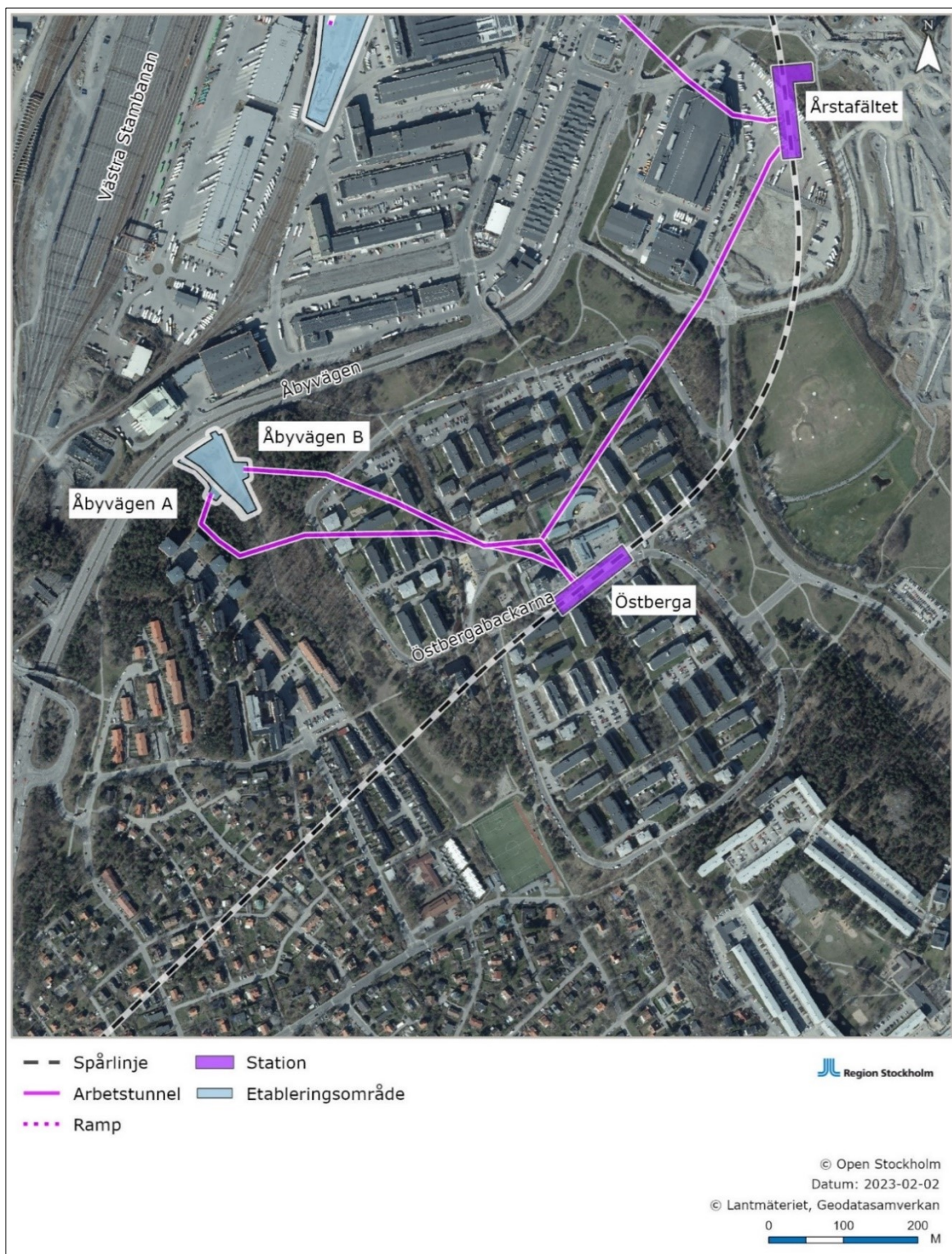
Figur23. Studerade arbetstunnlar och tillhörande etableringsytor för station Östberga. Spårlinje och arbetstunnlarnas sträckning är ungefärliga.
