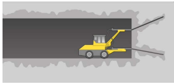
Steg 2: Injektering, betong sprutas in i borrhål och bergssprickor. När betongen stelnat bildas en tätning runt den blivande tunneln.
