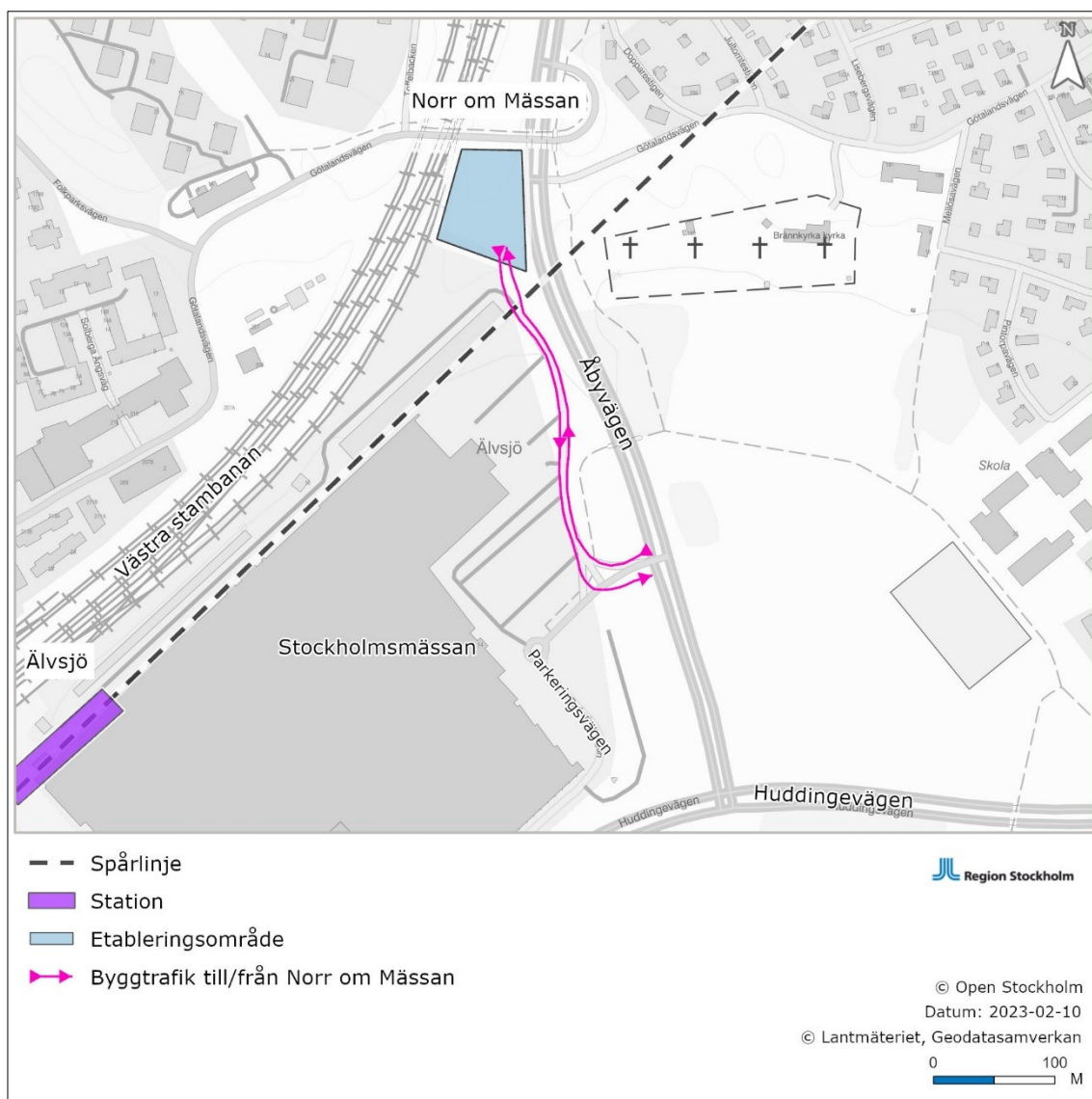
Figur 30. Möjliga transportvägar för alternativet Norr om mässan.
