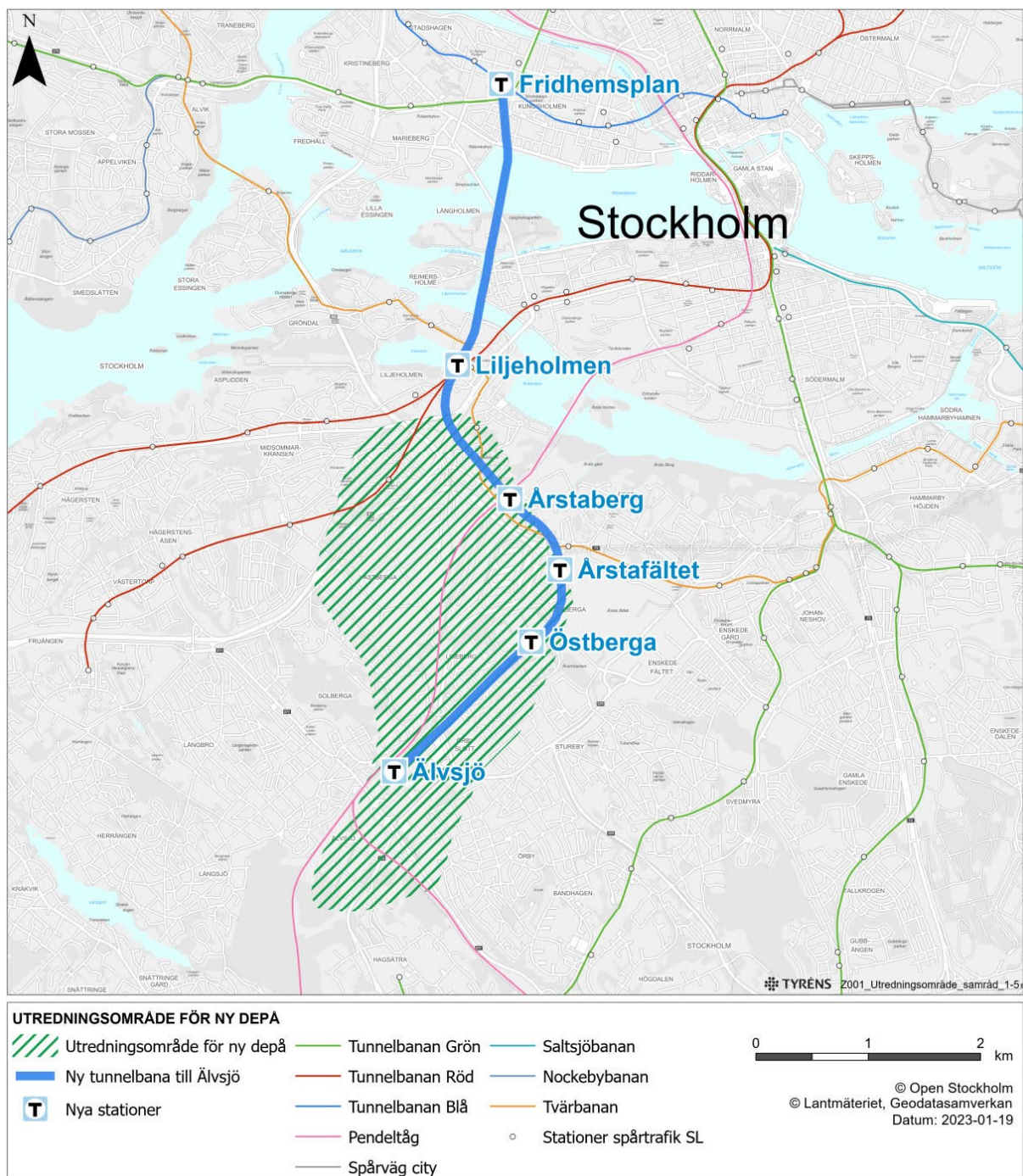
Figur 31. Utredningsområdet för en ny depå.
