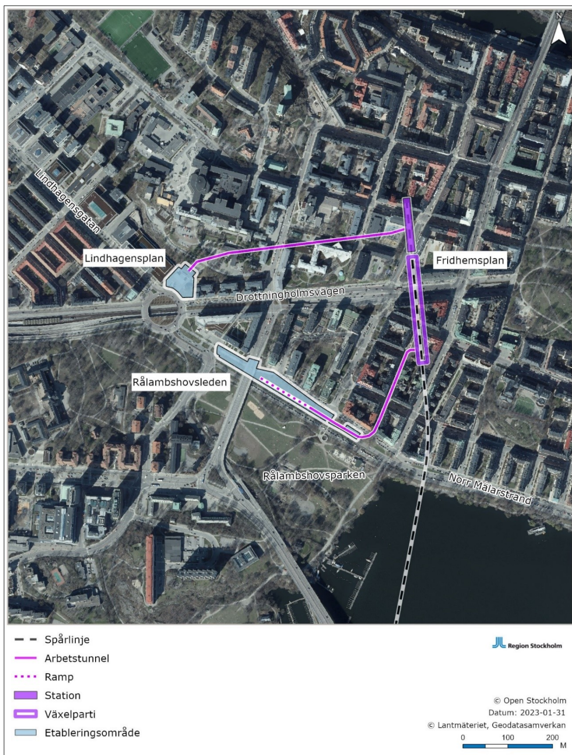
Figur 6. Studerade arbetstunnlar och tillhörande etableringsytor för station Fridhemsplan. Spårlinje och arbetstunnlarnas sträckning är ungefärliga.
