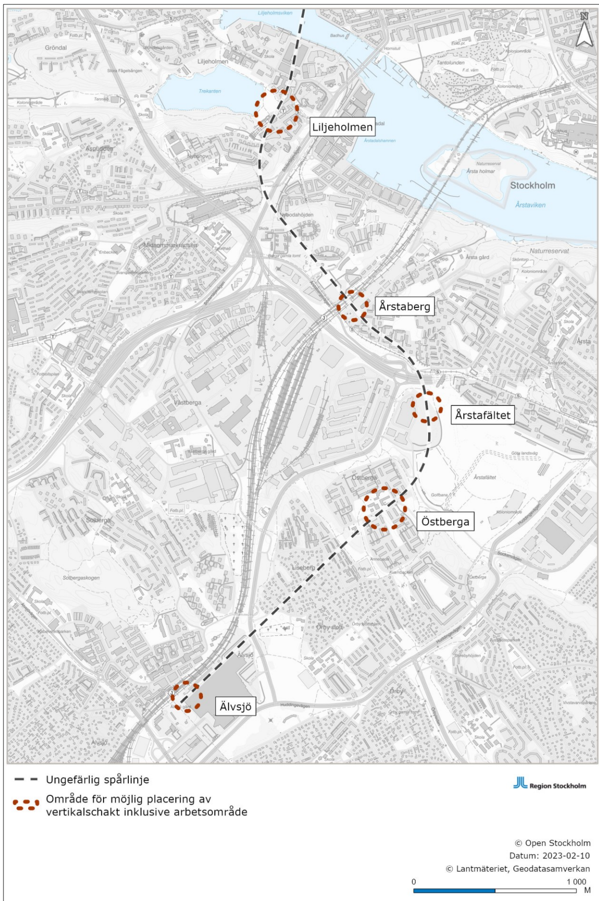
Figur 4. Områden som utreds för möjlig placering av vertikalschakt i Liljeholmen, Årstaberg, Årstafältet, Östberga och Älvsjö. Vid Fridhemsplan utreds inte denna möjlighet.
