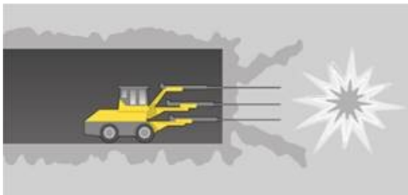
Steg 3: 1-5 meter långa hål borraras för sprängning och laddas sedan med sprängmedel. Sprängningen sker i etapper enligt ett bestämt mönster för att minimera vibrationerna.
