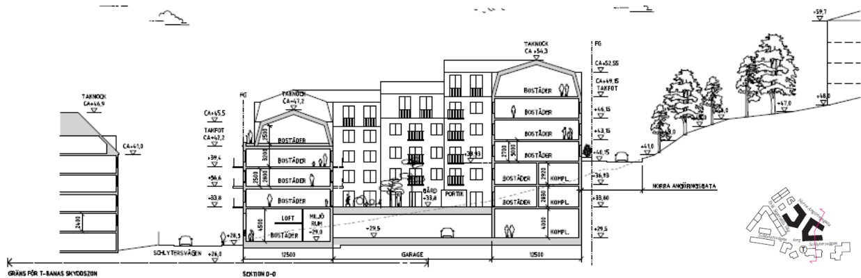
Sektion över Schlytersvägen vid Centrala delens östra del. Befintlig bebyggelse till vänster. Illustration: DinellJohansson
