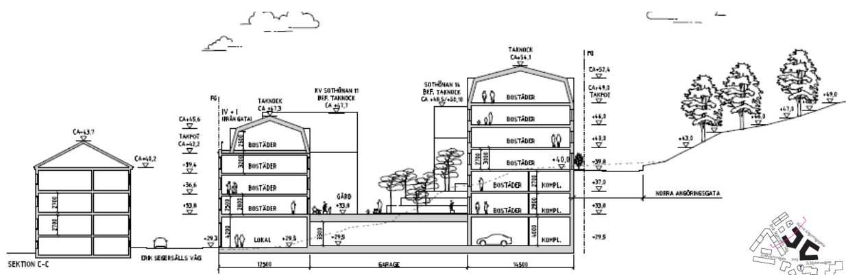
Sektion över Erik Segersälls väg vid Centrala delens västra del.. Befintlig bebyggelse till vänster. Illustration: DinellJohansson
