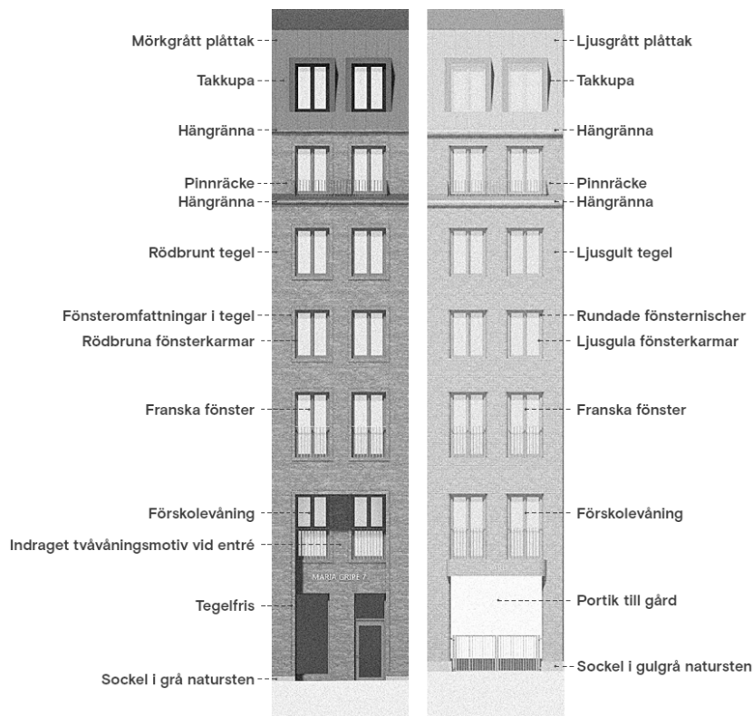
Fasadutsnitt för materialval, kulör och detaljer. (BSK)
