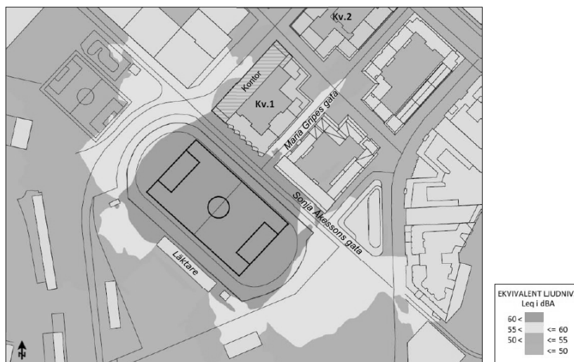
Beräknad ekvivalent ljudnivå under fotbollsmatch med herrseniorer med publik på läkare 1000 personer samt hejarklack. Ljudutbredning 1,5 meter över mark. (efterklang)
