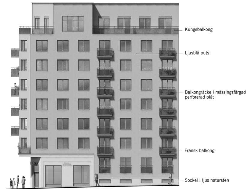
Fasadutsnitt som redovisar fasadindelning, materialval och detaljer. (AIX)
