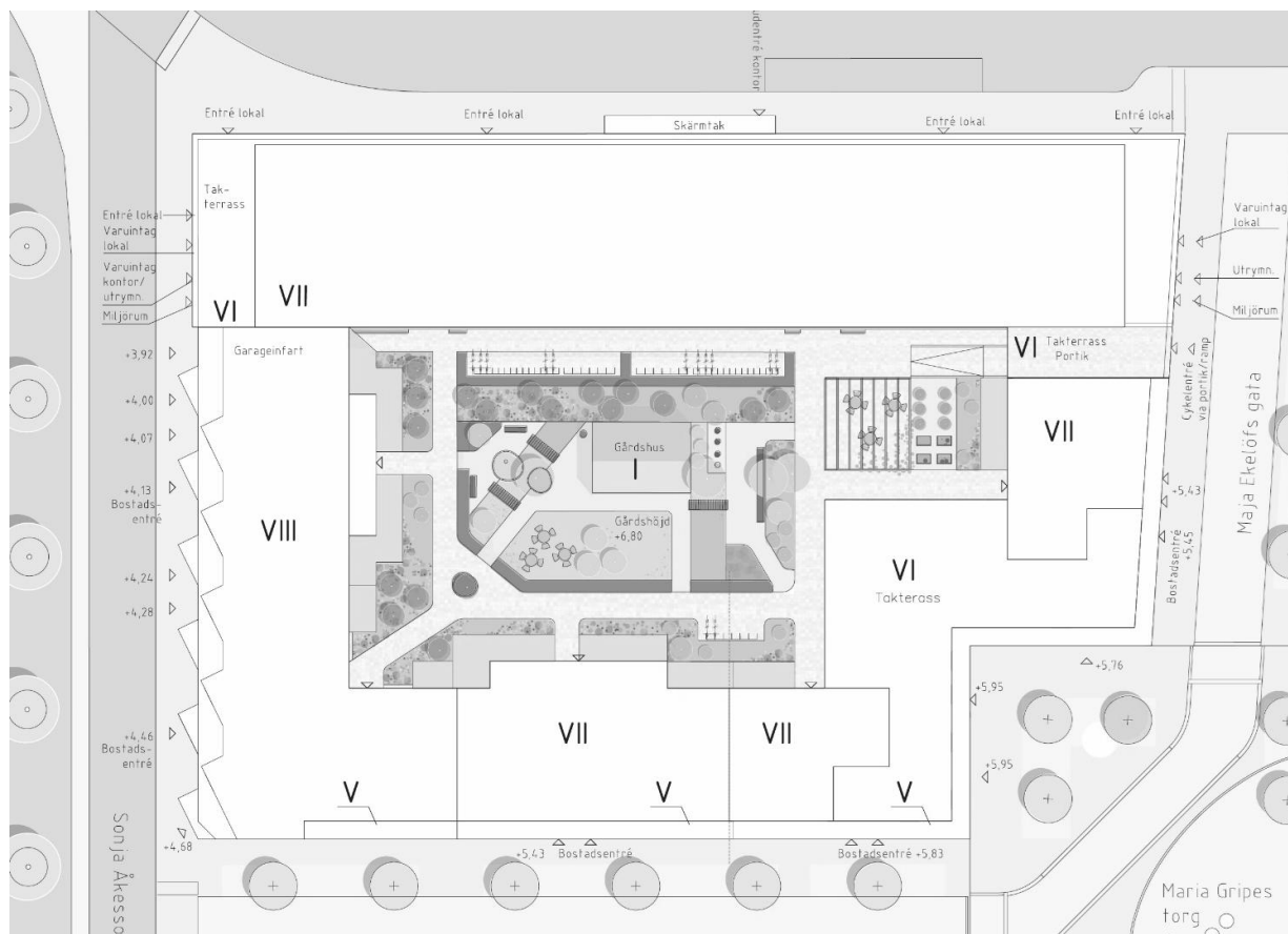
Illustrationsplan för kvarter 1. (Bjerking)
