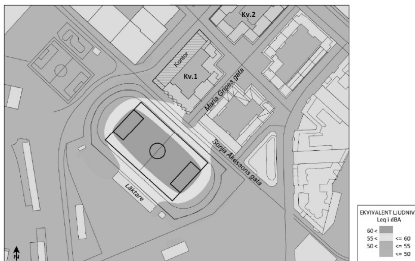
Beräknad ekvivalent ljudnivå under fotbollsträning med juniorer. Ljudutbredning 1,5 meter över mark. (efterklang)
