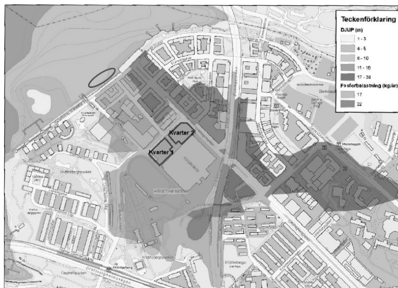
Avrinningsområde till skärbassäng vid Hornsbergsstrand. Placering av skärbassäng redovisas med röd ellips. (Bejrkning)
