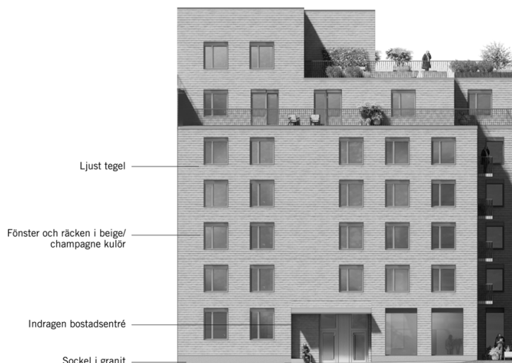
Fasadutsnitt som redovisar fasadindelning, materialval och detaljer. (AIX)
