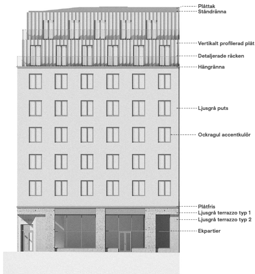
Fasadutsnitt för materialval, kulör och detaljer. (BSK)
