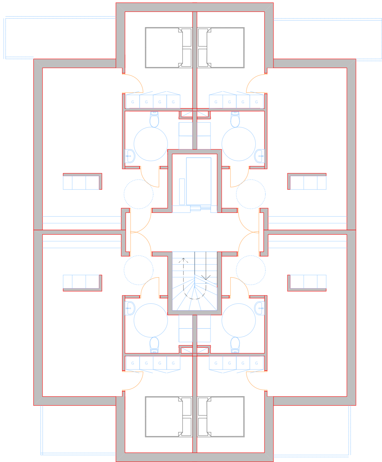
TYPPLAN 1:100
