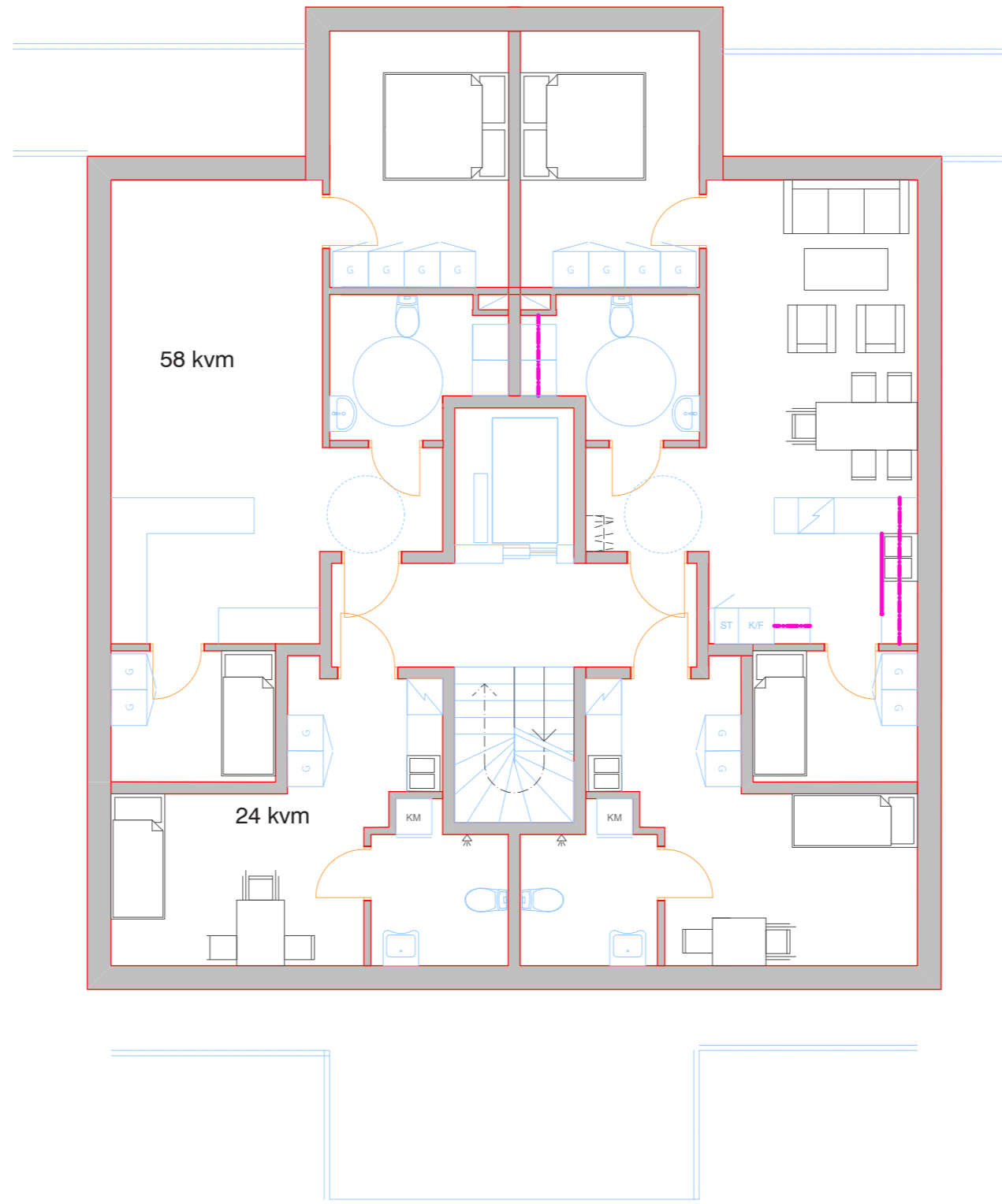
TAKPLAN - ALTERNATIV 02 1:100
