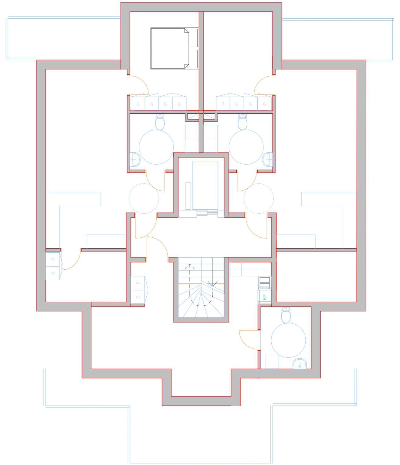
TAKPLAN - ALTERNATIV 01 1:100
