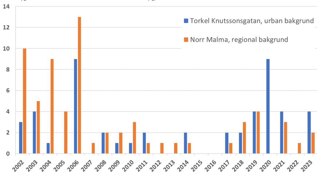
Figur 13. Trender för antal dygn med åttatimmars rullande medelvärde av ozon högre än normvärdet 120 µg/m 3 i urban och regional bakgrundsluft åren 2002–2023.
