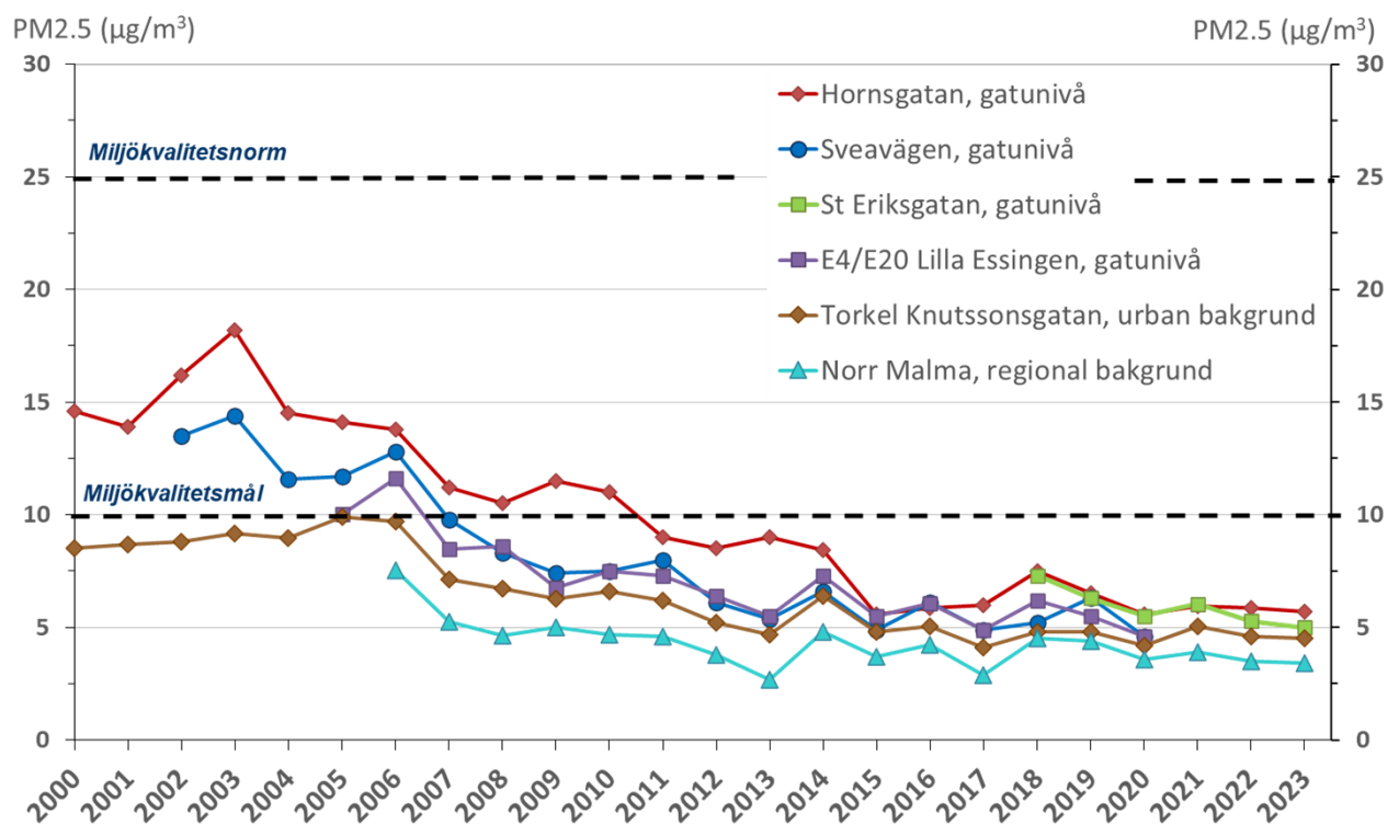
Figur 8. Trender för partiklar, PM2.5, årsmedelvärden under perioden 2000–2023 vid mätstationer i gatunivå samt i urban och regional bakgrundsmiljö.
