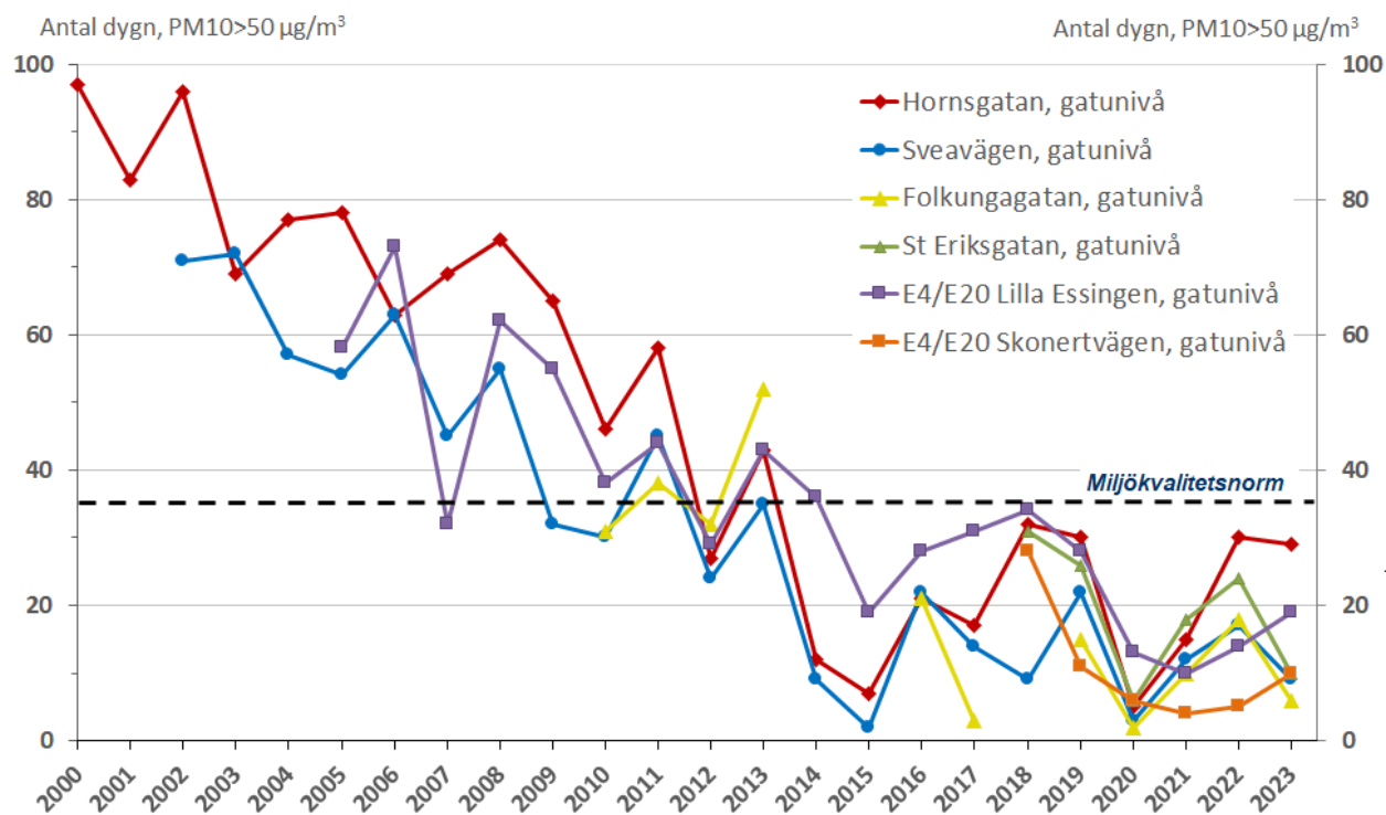
Figur 7. Trender för partiklar, PM10, antal dygnsmedelvärden högre än normvärdet 50 µg/m 3 för perioden 2000–2023 vid mätstationer i gatunivå. Maximalt antal tillåtna är 35 enligt miljökvalitetsnormen.
