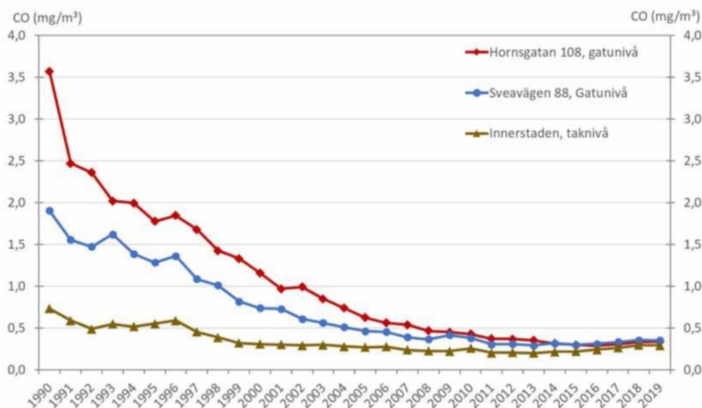
Figur 2. Trend för uppmätta årsmedelhalter av kolmonoxid åren 1990–2019 vid mätstationerna på Hornsgatan och Sveavägen. Halterna av kolmonoxid i taknivå är ett medelvärde av stationerna i taknivå på Hornsgatan och Sveavägen.
