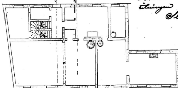
Plan of bottensvåningen
