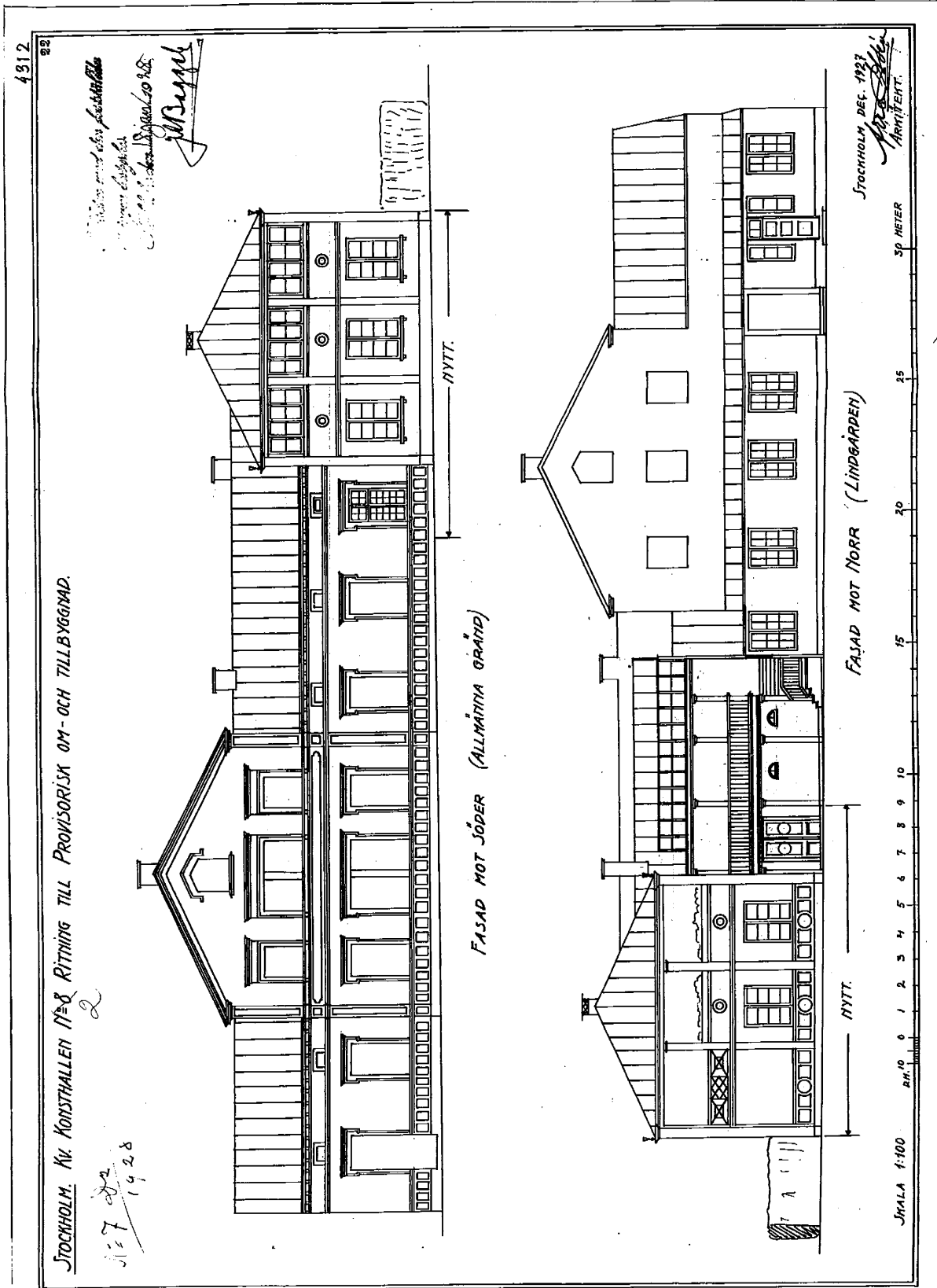
Tillbyggnad 1927, fasader. SBEx
