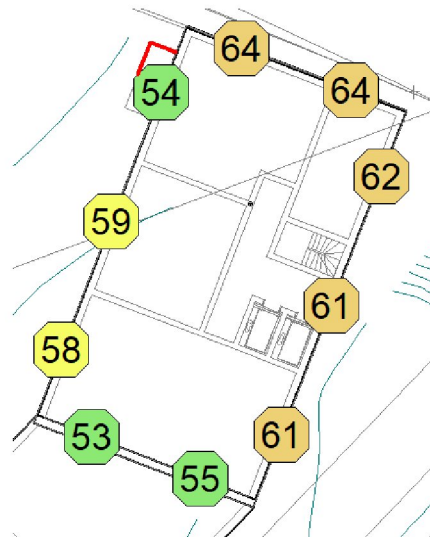
Figur 10 – Ekvivalenta ljudnivåer med skärmar i högdelen, våning 8-14. 7 berörda lägenheter.
