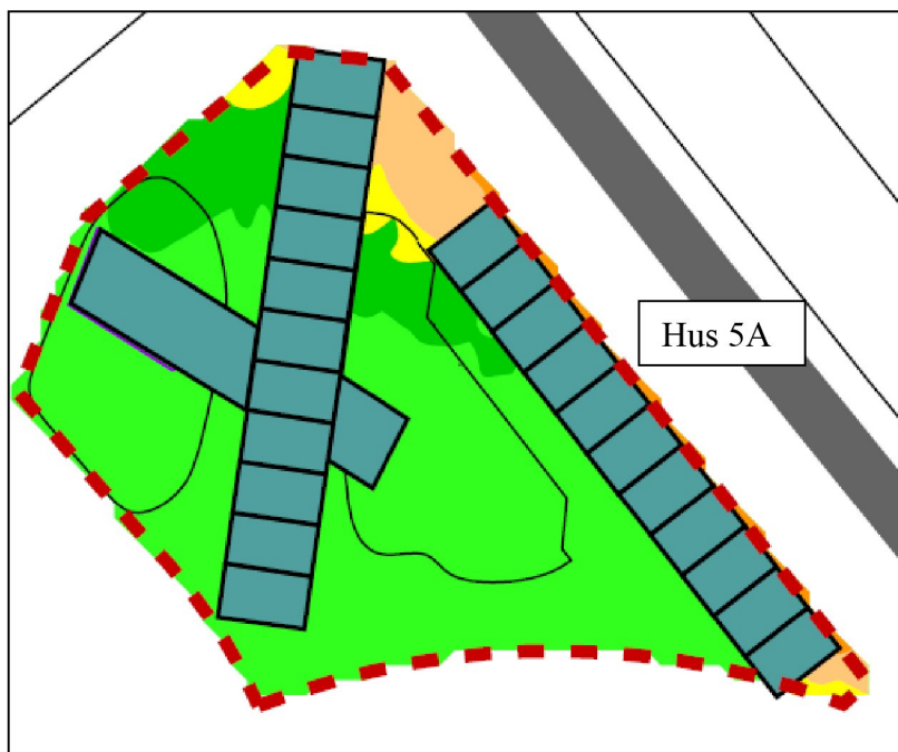
Bild 5 visar maximal ljudnivå från vägtrafik 2 meter över mark när del av förskolan placerats på mark. En stor del av förskolegården innehåller ljudkrav för maximal ljudnivå.
