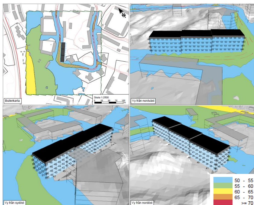
Dygnskvivalent ljudnivå, prognos 2030 (Cowi).
