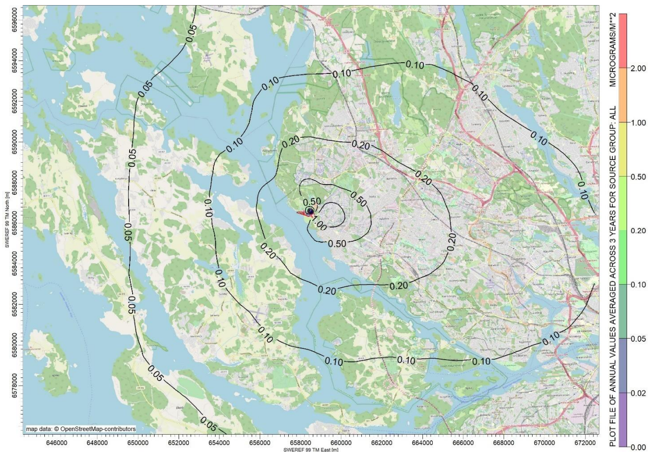
Figur 32. Deposition av nickel ( \mu\text{g}/\text{m}^2 )
