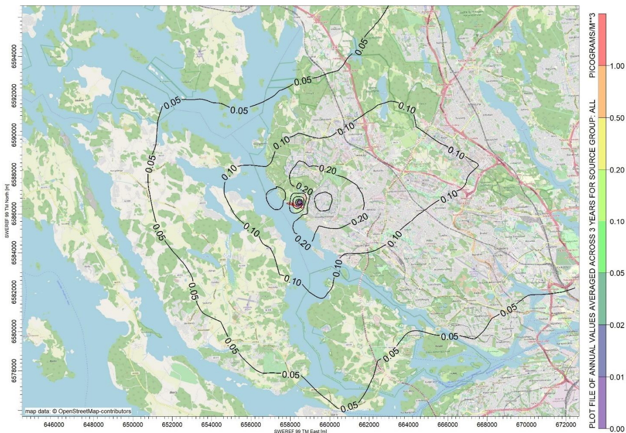
Figur 23. Kadmium som årsmedelvärden ( \text{pg}/\text{m}^3 )
