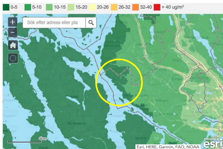
Figur 1. Bakgrundshalter av kvävedioxid som årsmedelvärde år 2015.
