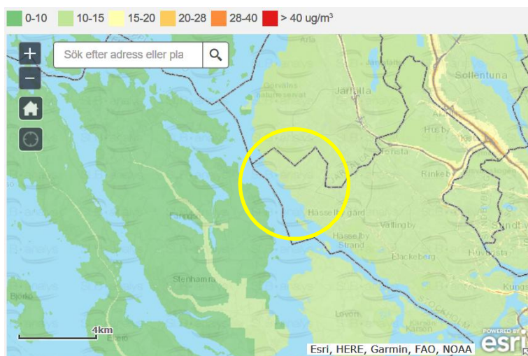
Figur 4. Bakgrundshalter av partiklar \text{PM}_{10} som medelvärden år 2015. Bakgrundshalterna av partiklar inom en radie på 3 km från den aktuella anläggningen ligger på omkring 0 – 15 \mu\text{g}/\text{m}^3 .
