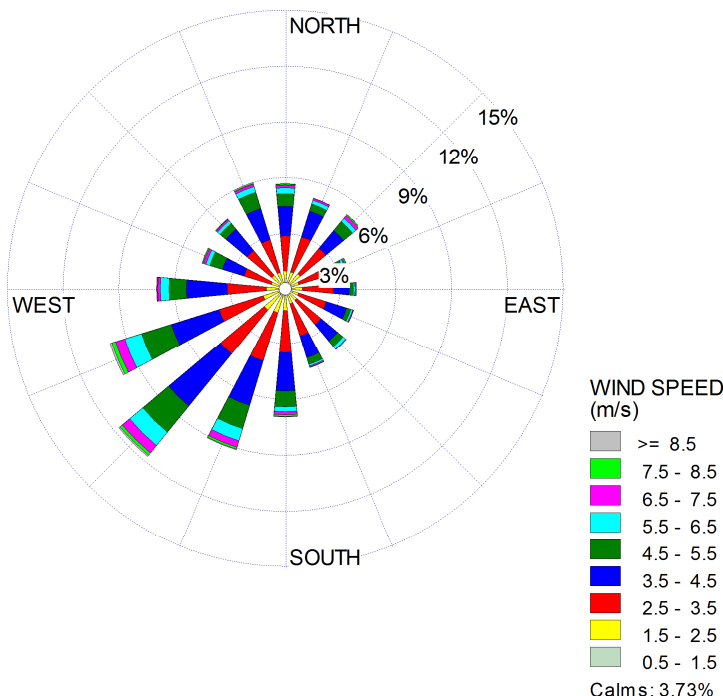
Figur 6. Vindros för meteorologiska data vid Lövsta åren 2015 - 2017
