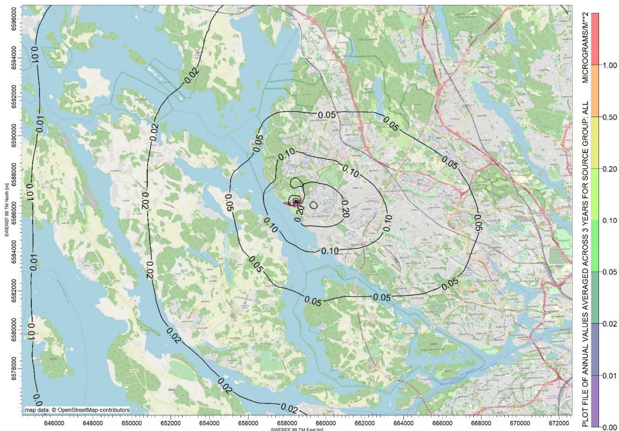
Figur 28. Deposition av arsenik ( \mu\text{g}/\text{m}^2 )
