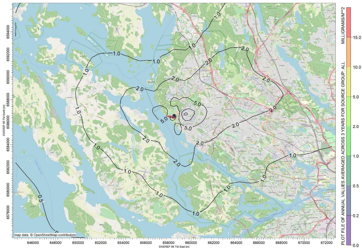
Figur 26. Deposition av kväve (mg/m 2 )
