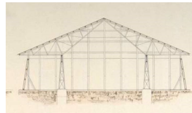
Ovan: Bild 50: Ritningar på konstruktionen på det nu rivna kolhuset i Gävle, 1892. Källa: Gävle kommun.
