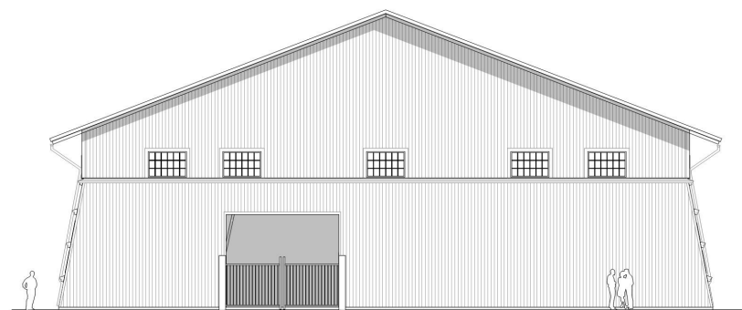
Bild 20: Fasadritning mot nordost. Källa: Koncept.
