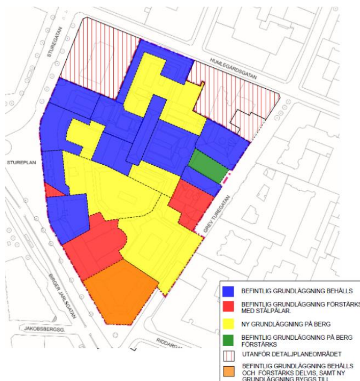
Kartan visar grundläggningsåtgärder inom planområdet.
