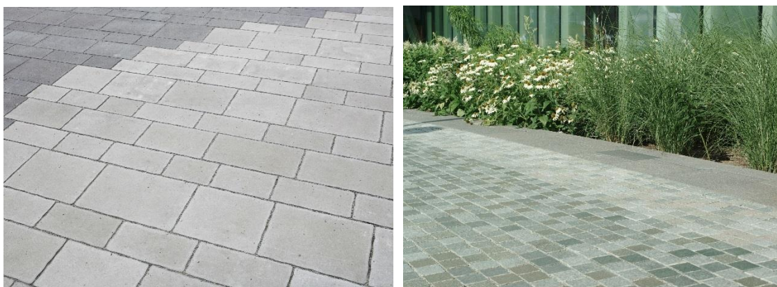
Figur 6 Stenplattor med avstånd för infiltration. Källa: grus.nu & arctic-kvartsit.se .
