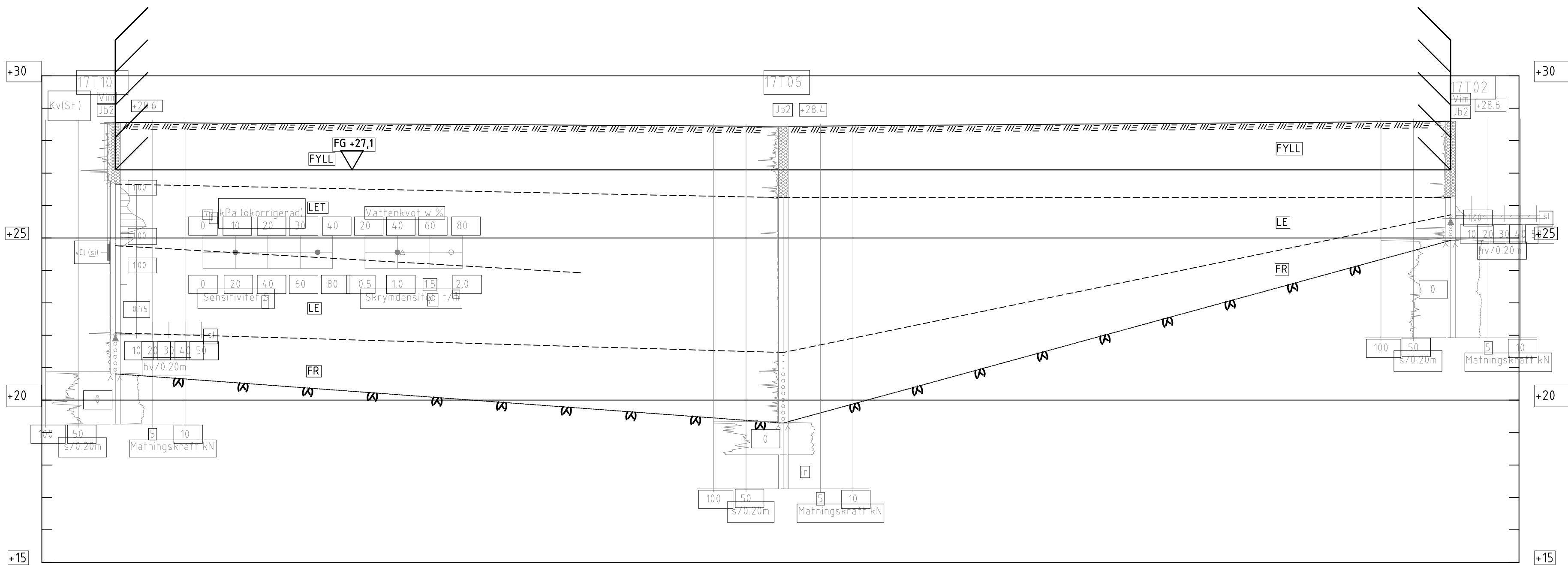
SEKTION E-E
