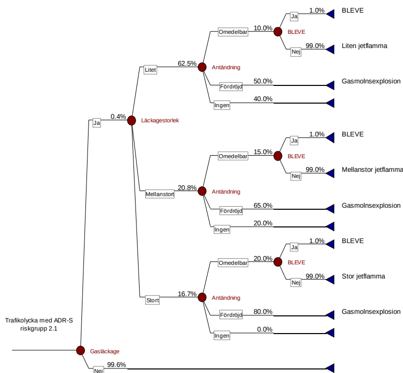
Figur 15. Händelsetråd med sannolikheter för ADR-S klass 2.1.
