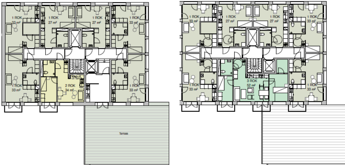
Figur 5. Planlösning hus C. Plan 5 (t.v.) och plan 6–15 (t.h.).
