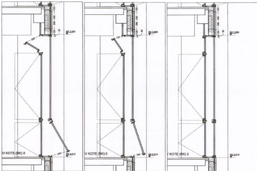
Figur 9. Exempel på tekniska åtgärd med specialfönster. Fönstret möjliggör vädning i nedkant, se bild till vänster och i mitten, utan att ljudmiljön inomhus försämras avsevärt.
