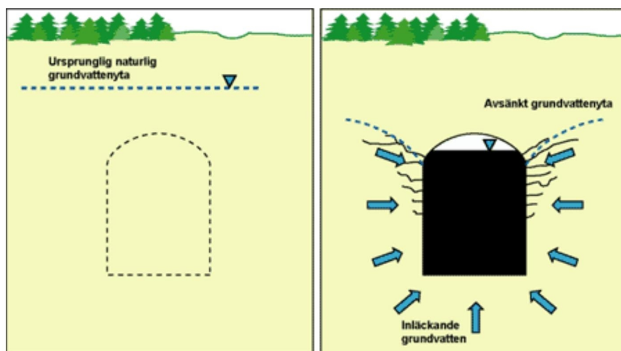
Figur 2: Lagringsprincip i ett oljebergtrum (Bild: SGU)
