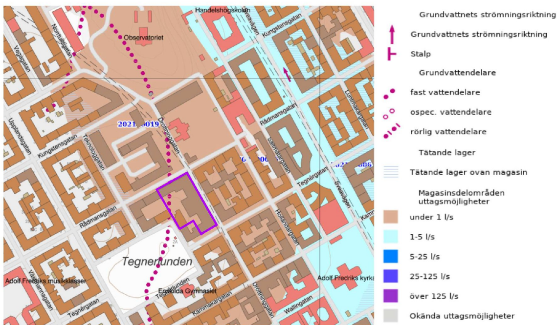
Figur 6. Grundvattenmagasin enligt SGU:s kartvisare. (SGU, 2019).
