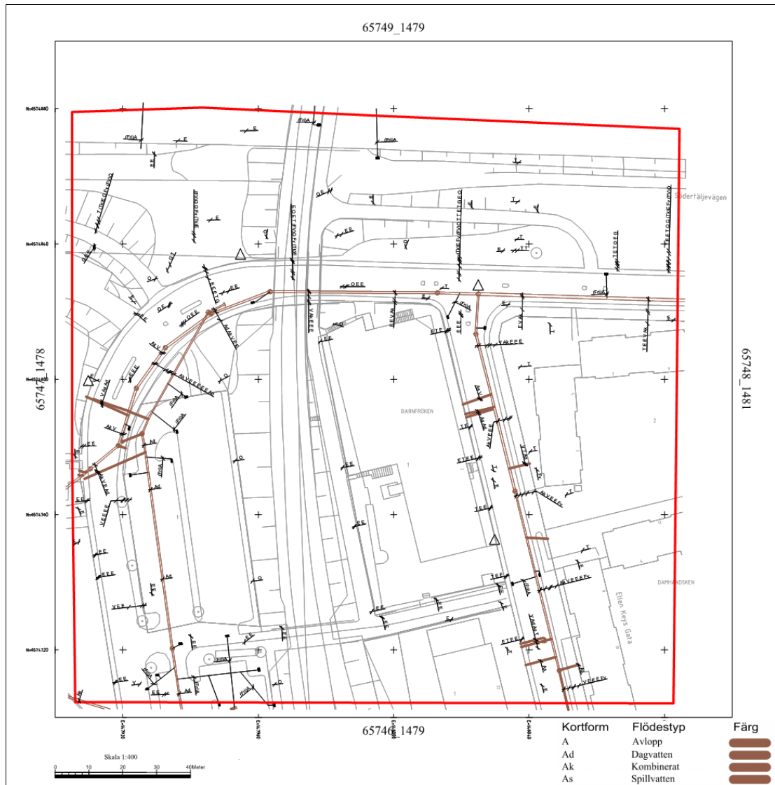
Figur 4. Samlingskartan visar dagvattnets anslutning till det kombinerade nätet (Samlingskarta, Trafikkontoret Stockholm Stad)
