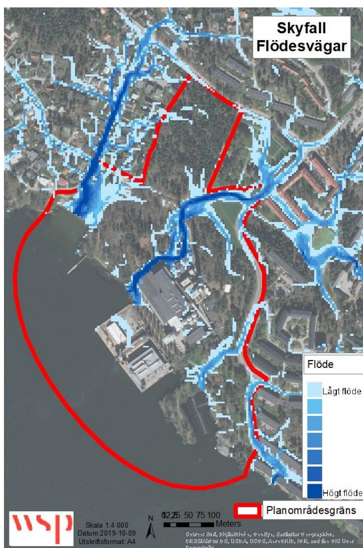
Skyfallsmodellering, flödesvägar. Avvikelse kan förekomma. (WSP)
