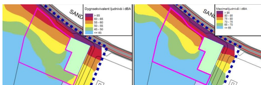
Dygnsekvivalent ljudnivå till vänster och maximal ljudnivå till höger 1,5 m över mark vid den norra förskolegården utan åtgärder. Avvikelser kan förekomma (Structor)
