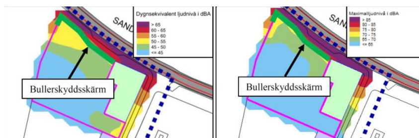
Dygnsekvivalent ljudnivå till vänster och maximal ljudnivå till höger 1,5 m över mark vid den norra förskolegården med en 2 m hög bullerskyddsskärm (grön linje) längs Sandviksvägen. Avvikelser kan förekomma (Structor)
