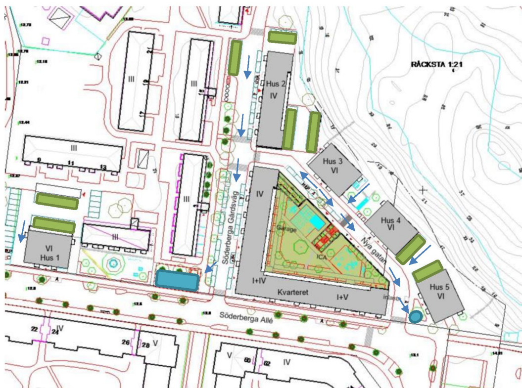
Figur 5. Föreslagna LOD-lösningar för planområdet. Gröna rektanglar markerar lokaliseringspunkter för parkeringsplatser försedda med genomsläpplig betongarmering och blåa rektanglar avser placering av nedsänkta regnväxtbäddar.
