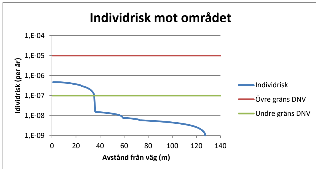
Figur 10. Individrisken som en funktion av avståndet från Örbyleden.
