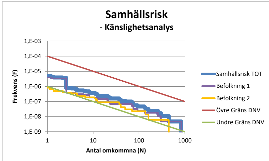
Figur 15. Samhällsrisk i känslighetsanalys.
