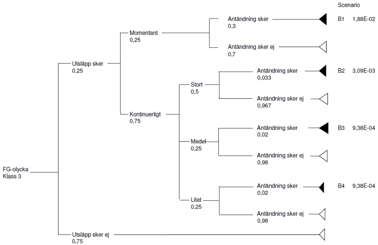
Figur A.2.3. Händelsetråd över farligt godsolycka med klass 3.
