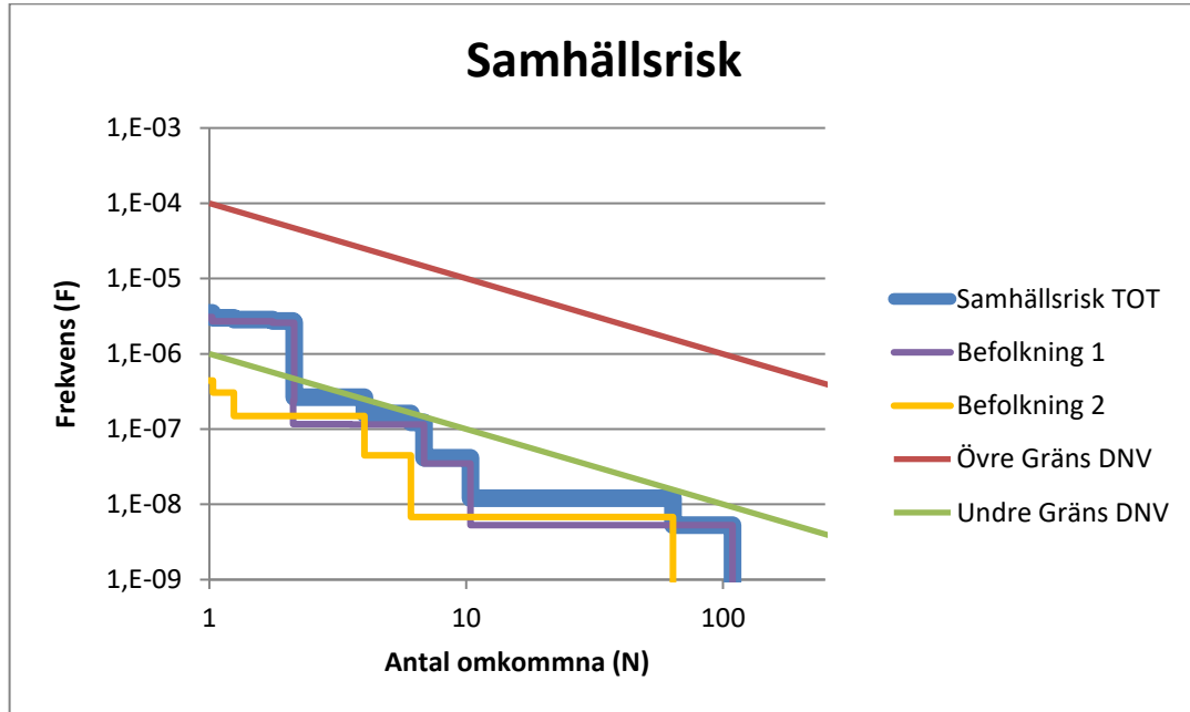
Figur 12. Samhällsrisik för planområdet utmed Örbyleden.
