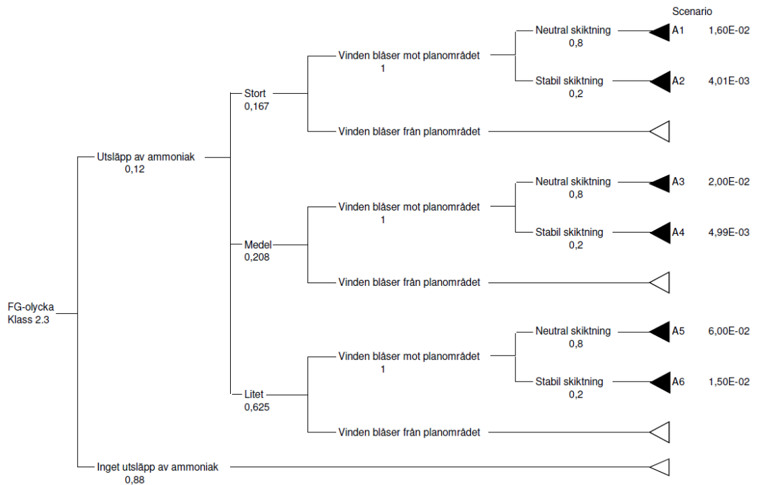
Figur A.2.2. Händelsetråd över farligt godsolycka med klass 2.3.
