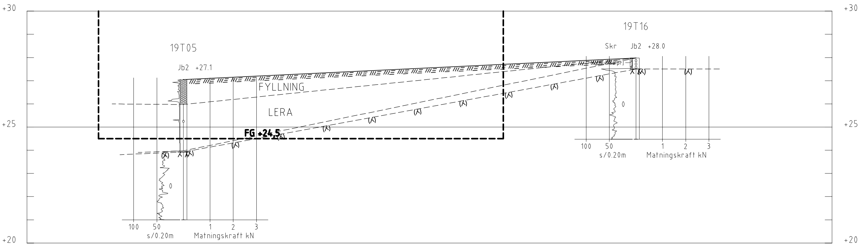
SEKTION G-G 1: 100
