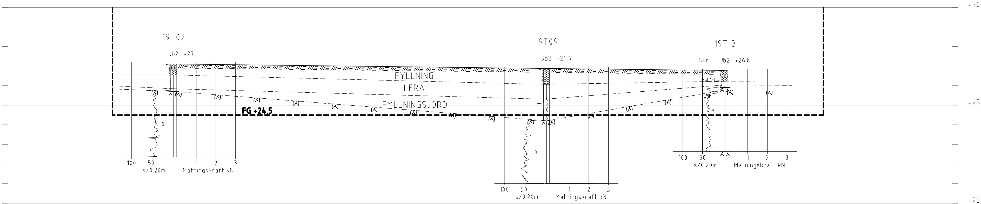
SEKTION D-D 1: 100
