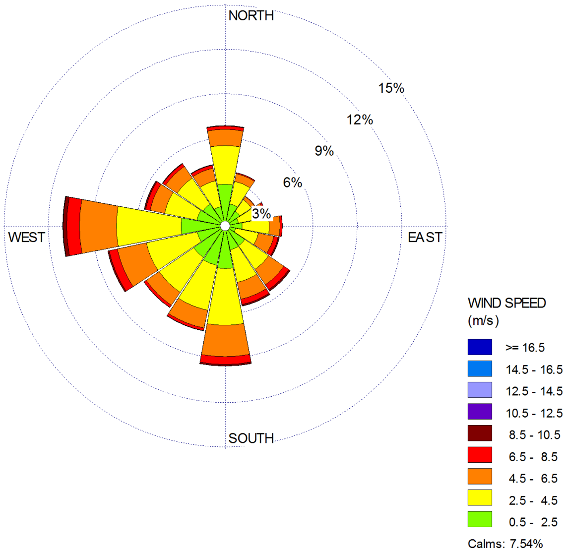
Figur 8-1: Vindros för hela året , Bromma flygplats 1986-2015. Medelvind 3.32 m/s.
