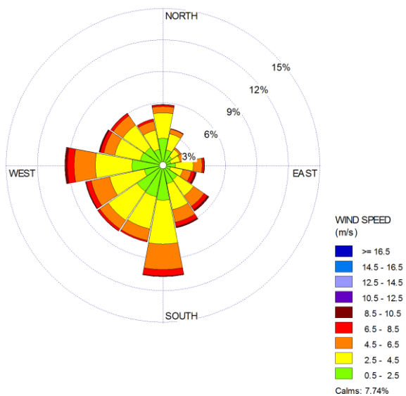
Figur 8-4: Vindros för hösten (september-november), Bromma flygplats 1986-2015. Medelvind 3.25 m/s.
