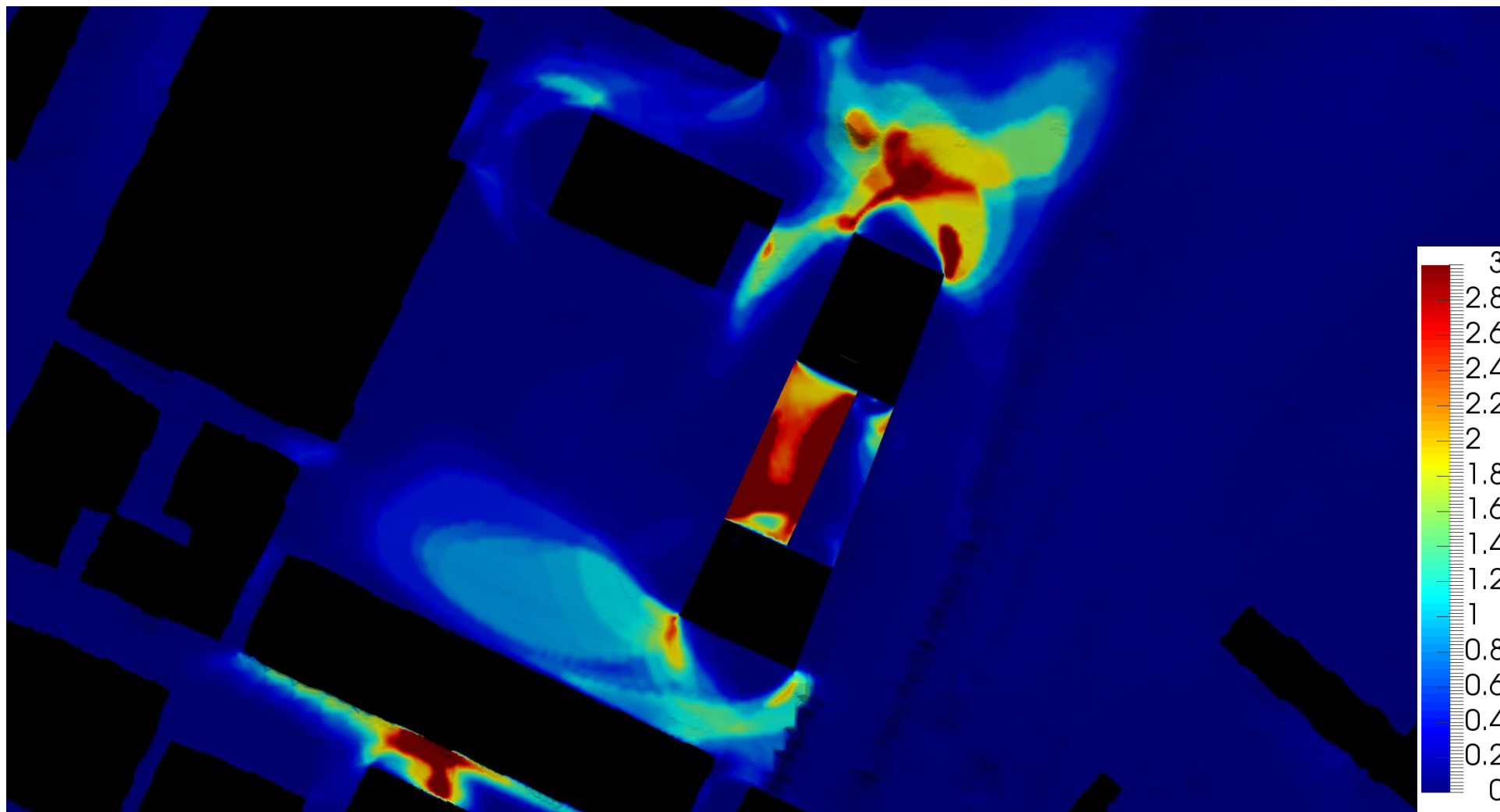
Figur 9-2. Procent av tiden som vindens hastighet överstiger 5 m/s, på 2 m höjd över marken. Sammanvägning av alla vindriktningar.
