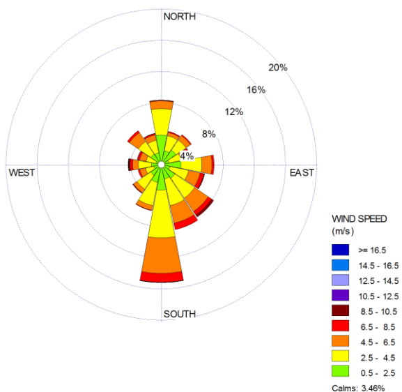
Figur 8-6: Vindros vid regn och duggregn , Bromma flygplats 2004-2015. Medelvind 3.51 m/s.
