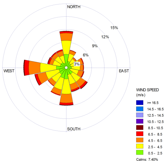
Figur 8-2: Vindros för våren (mars-maj), Bromma flygplats 1986-2015. Medelvind 3.41 m/s.
