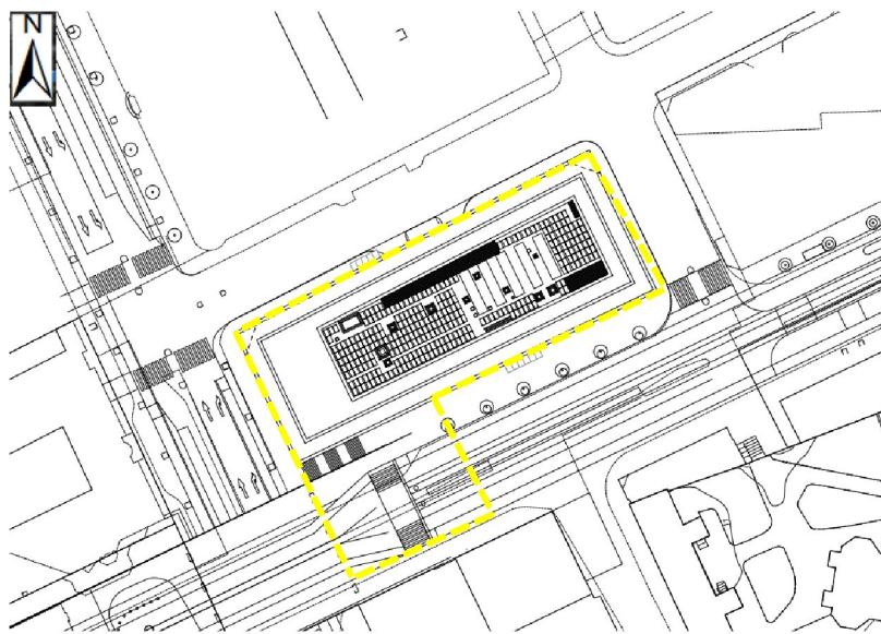
Figur 2. Situationsplan för området efter omdaning 1 med utredningsområdet markerat med gul streckad linje.
