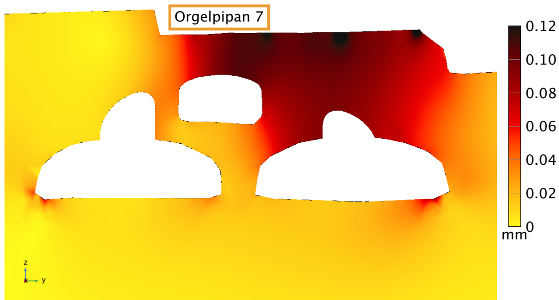
Figur 17: Snittplan genom RZ2. Total deformation i RZ2 vid pålastning om tre våningar [m].
