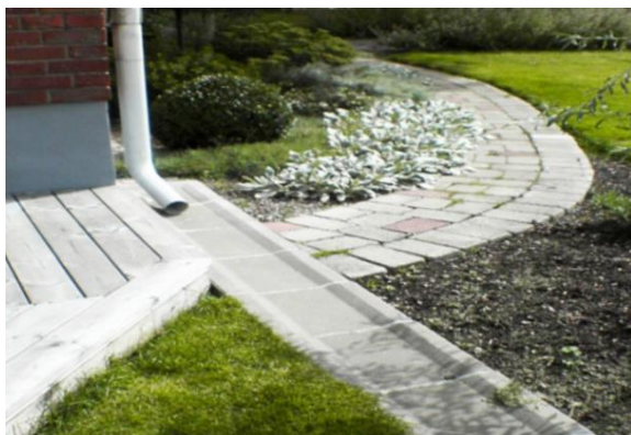
Figur 6-6. Exempel på stuprörsutkastare och dagvattenränna (SVU, 2014).
