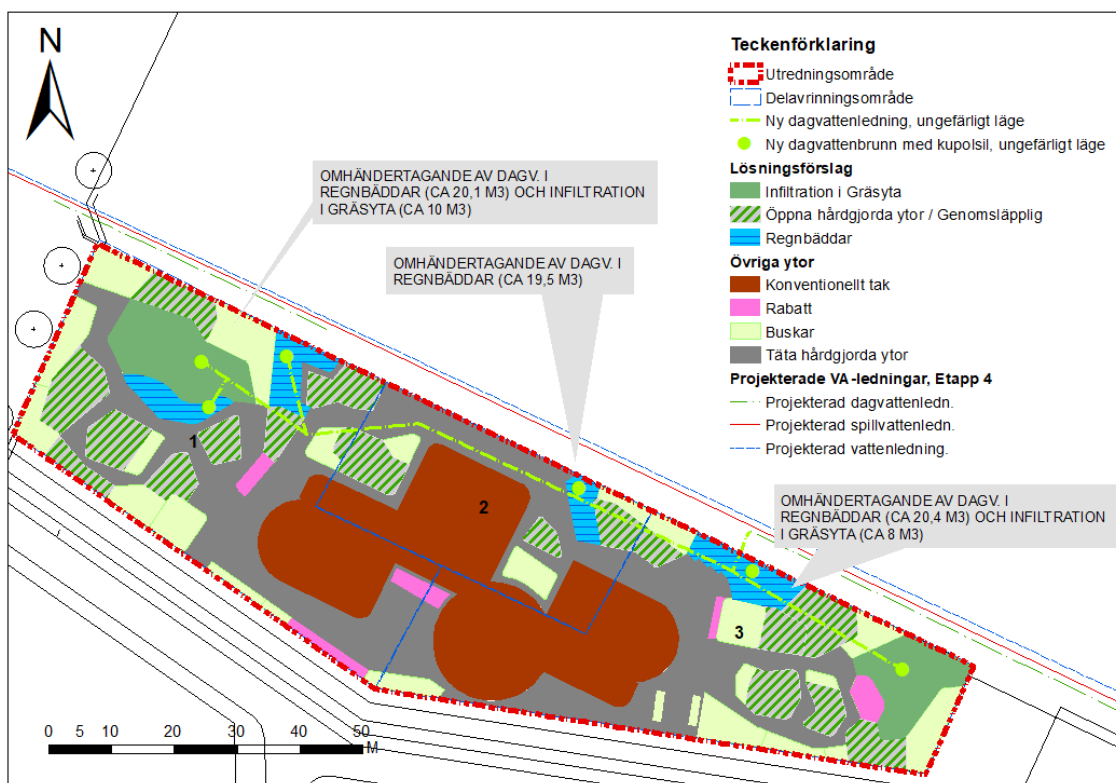
Figur 6-12. Lösningförslag för hållbar dagvattenhantering i utredningsområde, alternativ 2.
