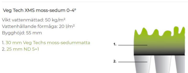
Figur 6-9. Principritning för utformning av gröna tak (VegTech, 2019).
