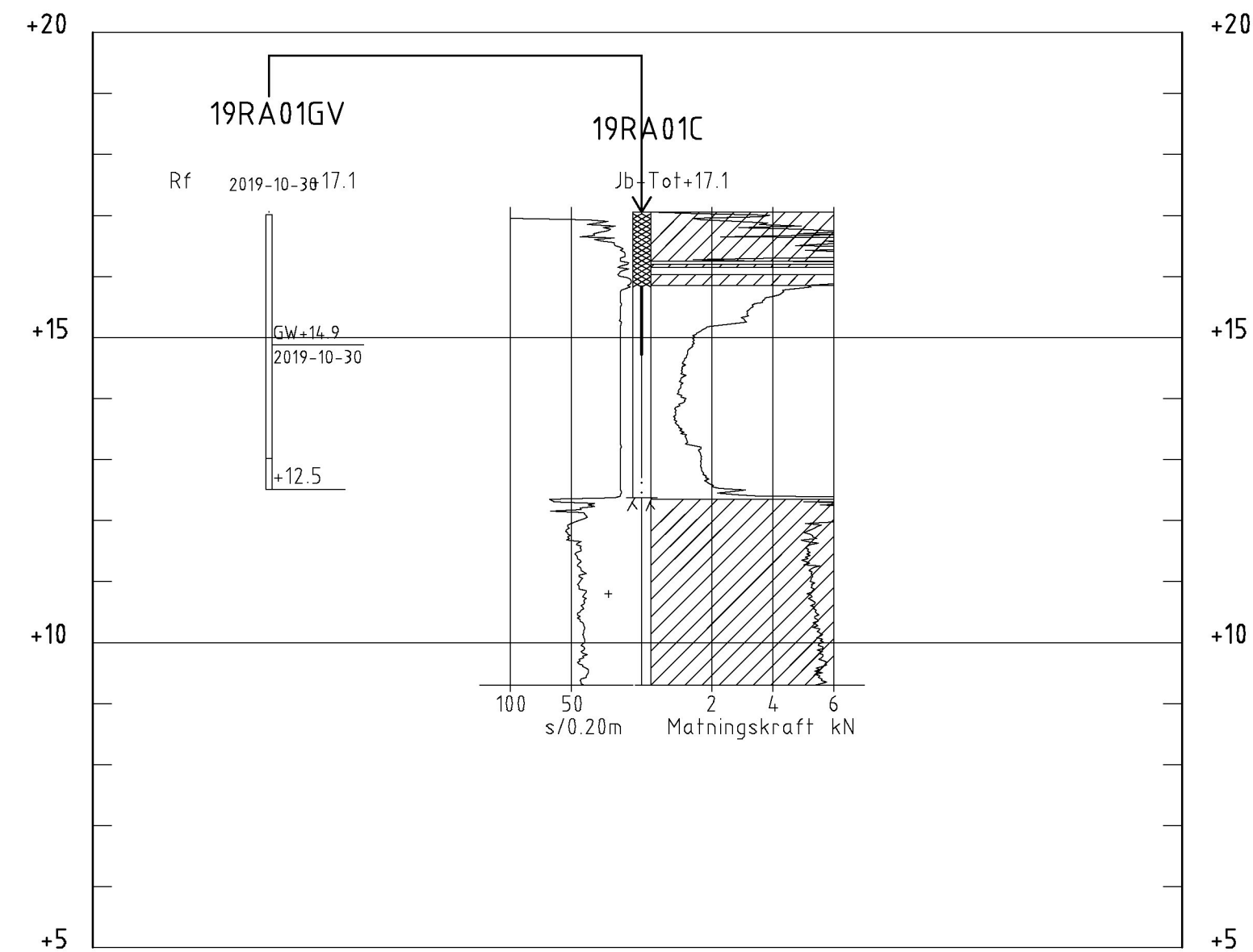
SEKTION C-C 1: 100
