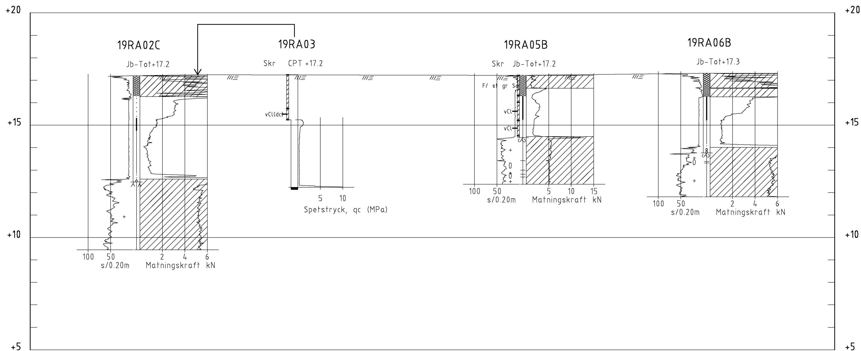
SEKTION B-B 1: 100
