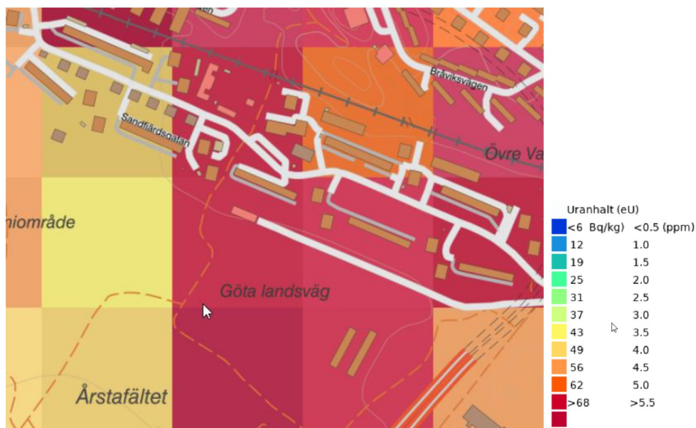
Figur 4. Uranhaltkarta, sgu.se
