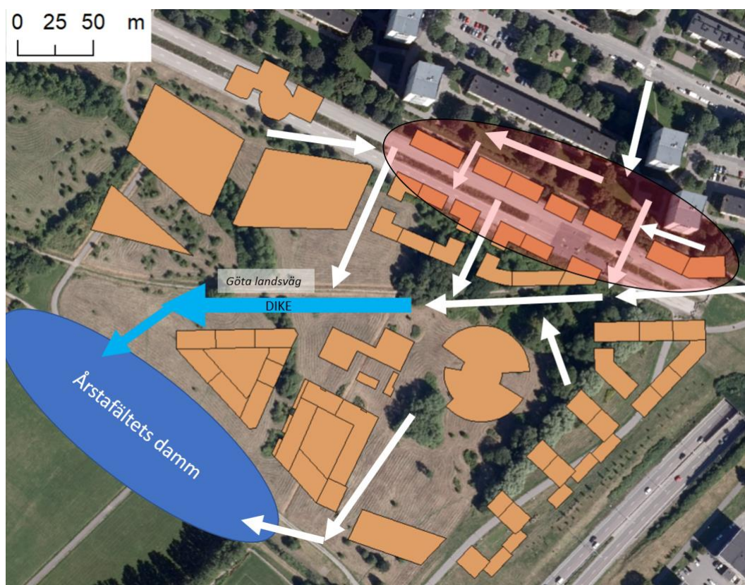
Figur 5. Skyfallsåtgärder inom Årstafältets Etapper 4a och b. Skyfallsvatten leds via dike till dammen. Höjdsättning är anpassad för att kunna avleda skyfallsvattnet till dammen på ett hållbart sätt. Vita pilar motsvarar önskat flödesriktning. I det röda området har det funnits utmaningar med att få till rätt höjdsättning på grund av platsbrist.
