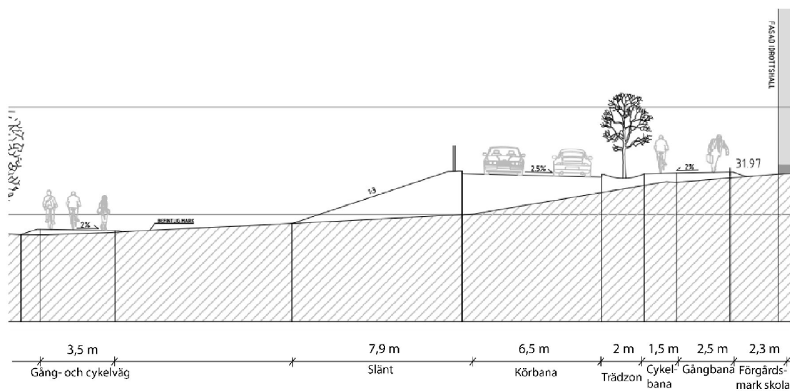
Figur 11. Sektionssnitt 2.
