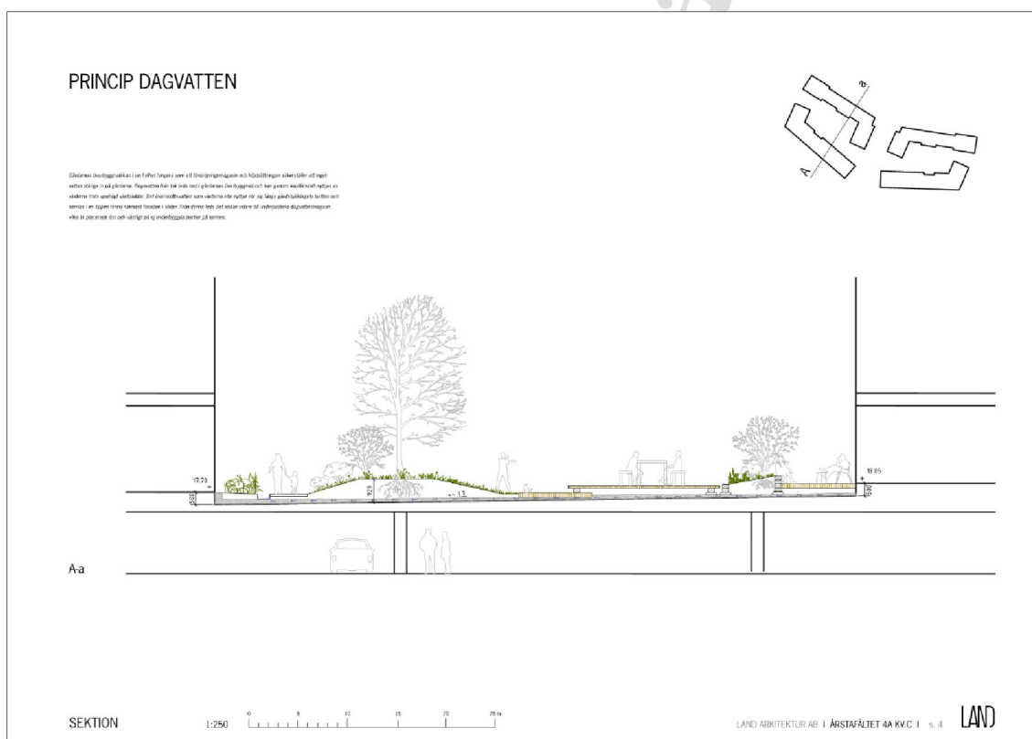
Figur 9-1. Exempelskiss på föreslagna dagvattenlösningar, inklusive makadamlager med ovanliggande planteringar och genomsläppliga ytor. I skissen är dagvattenränna placerad längs södra fasaden. Placerar ränna enligt skiss behöver den nedre delen av närliggande byggnads fasad skyfallssäkras. Det behöver också säkerställas en tillräcklig nivåskillnad mellan färdigt golv och ränna för att undvika att vatten i en översvämningssituation tränger in genom exempelvis portar. Skiss erhållen från LAND Arkitektur AB 2020-02-19.
