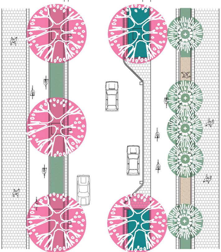
Figur 21: Typsektion och planutsnitt för gatuträd och ytskikt för sekvens 2 (mellan Nystadsgatan och Norgegatan). Likvärdig utformningsprincip som sekvens 1, men med andra arter
