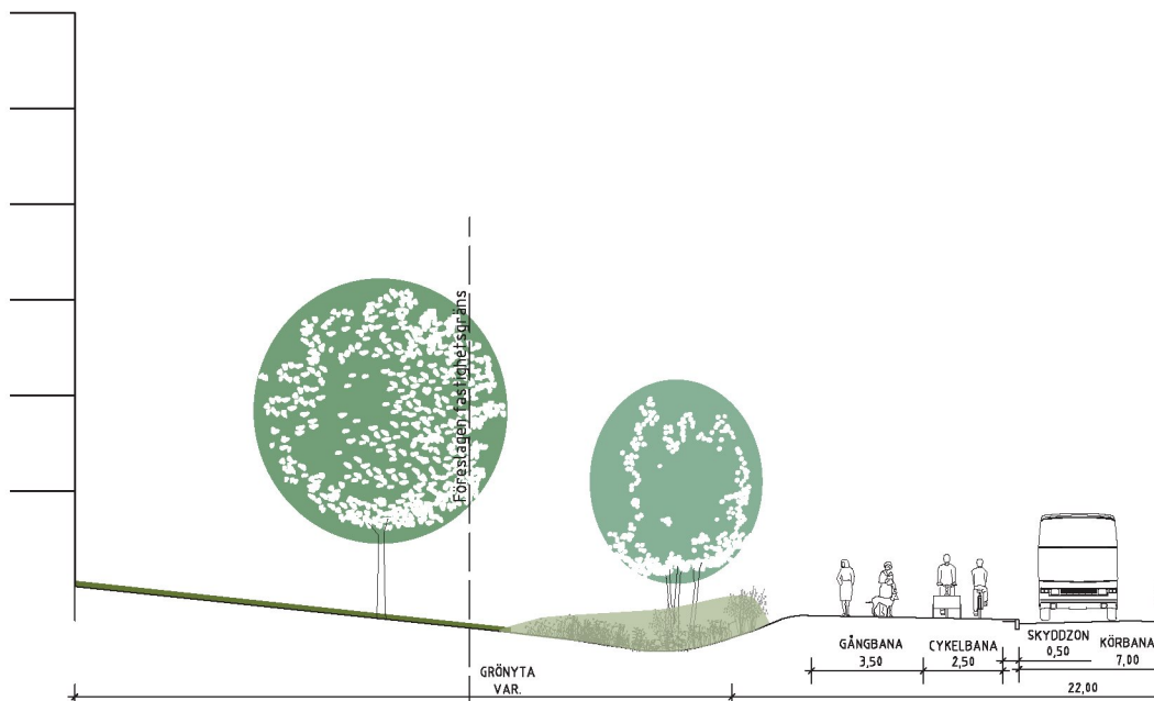
Figur 51: Sektion A-A, dagvattenstråket på västra sidan av Norgegatan. Dike med biobäddar utmed Norgegatan kan ta hand om regnvatten.
