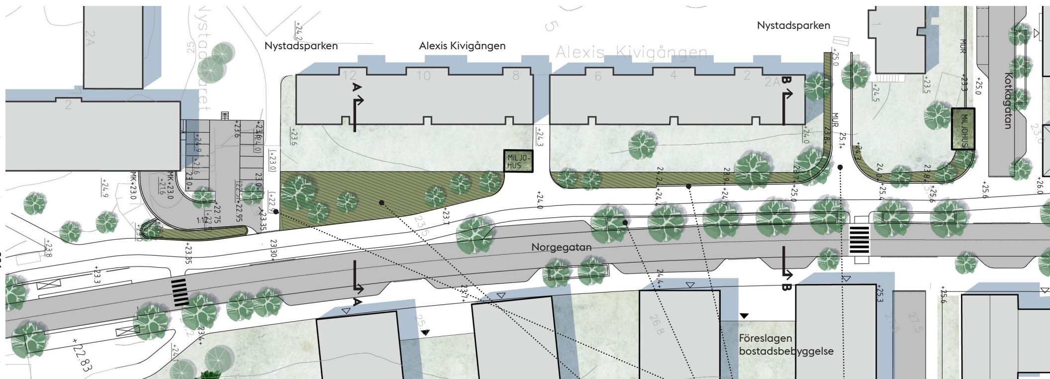
Figur 53: Västra Norgegatan illustrationsplan, Skala 1:800
