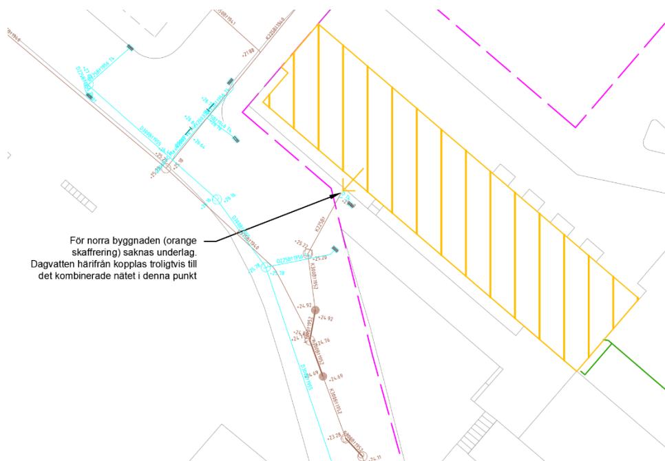
Figur 11 Översikt över dagvattenledningar för norra byggnaden. Underlag från SSSB saknas men dagvatten antas ledas till kombinerad ledning
