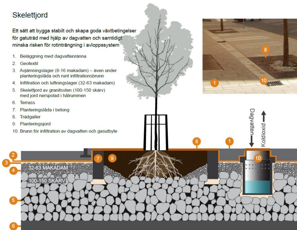
Figur 30 Principskiss för skelettjord. (Källa: Stockholm stad Trafikkontoret)
