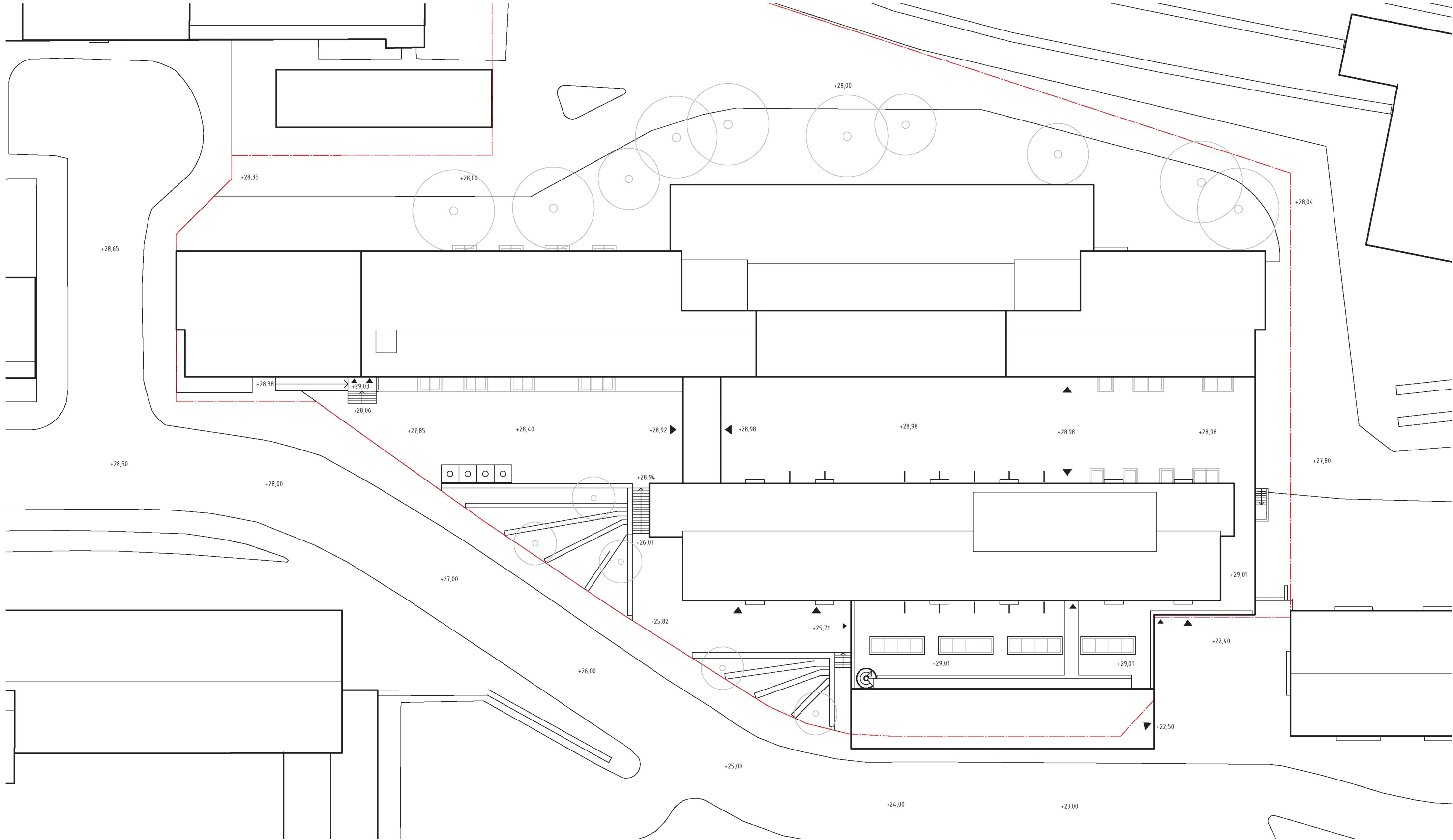
Situationsplan – Bebyggelse
