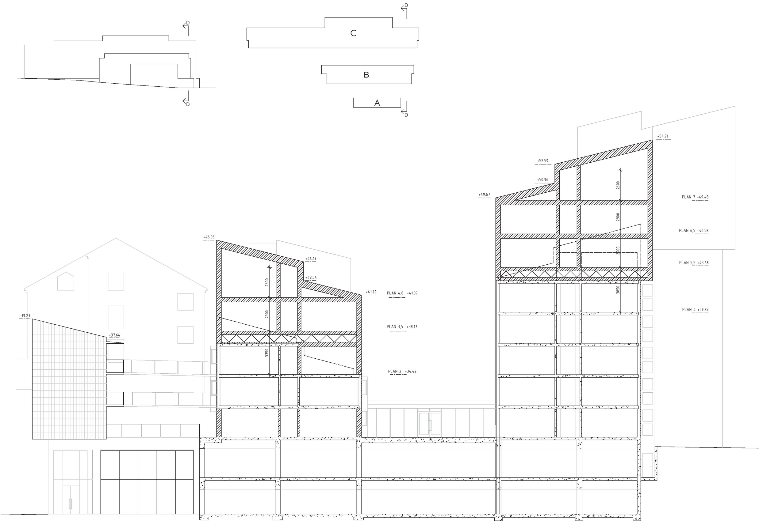
Sektion D-D
