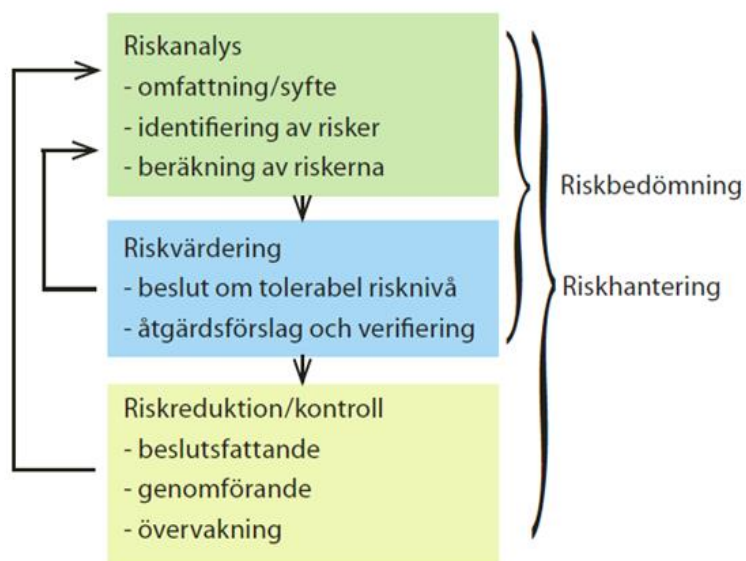
Figur 3. Riskhanteringsprocessen. Källa: [7].
