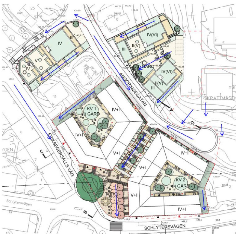
Utdrag från dagvattenutredningen som visar principen för skyfallshantering. Illustration Structor
